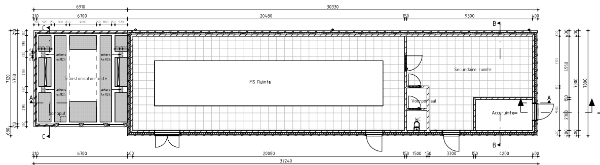
Plattegrond
