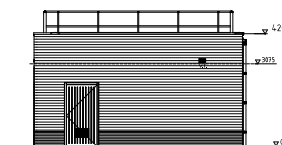
Rechter zijgevel
