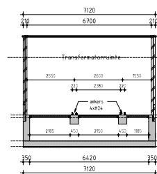
Doorsnede C-C
