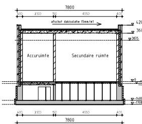
Doorsnede B-B
