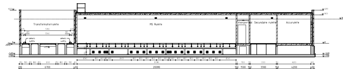
Doorsnede A-A
