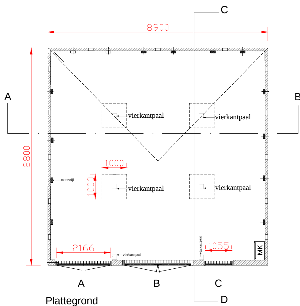
Plattegrond
