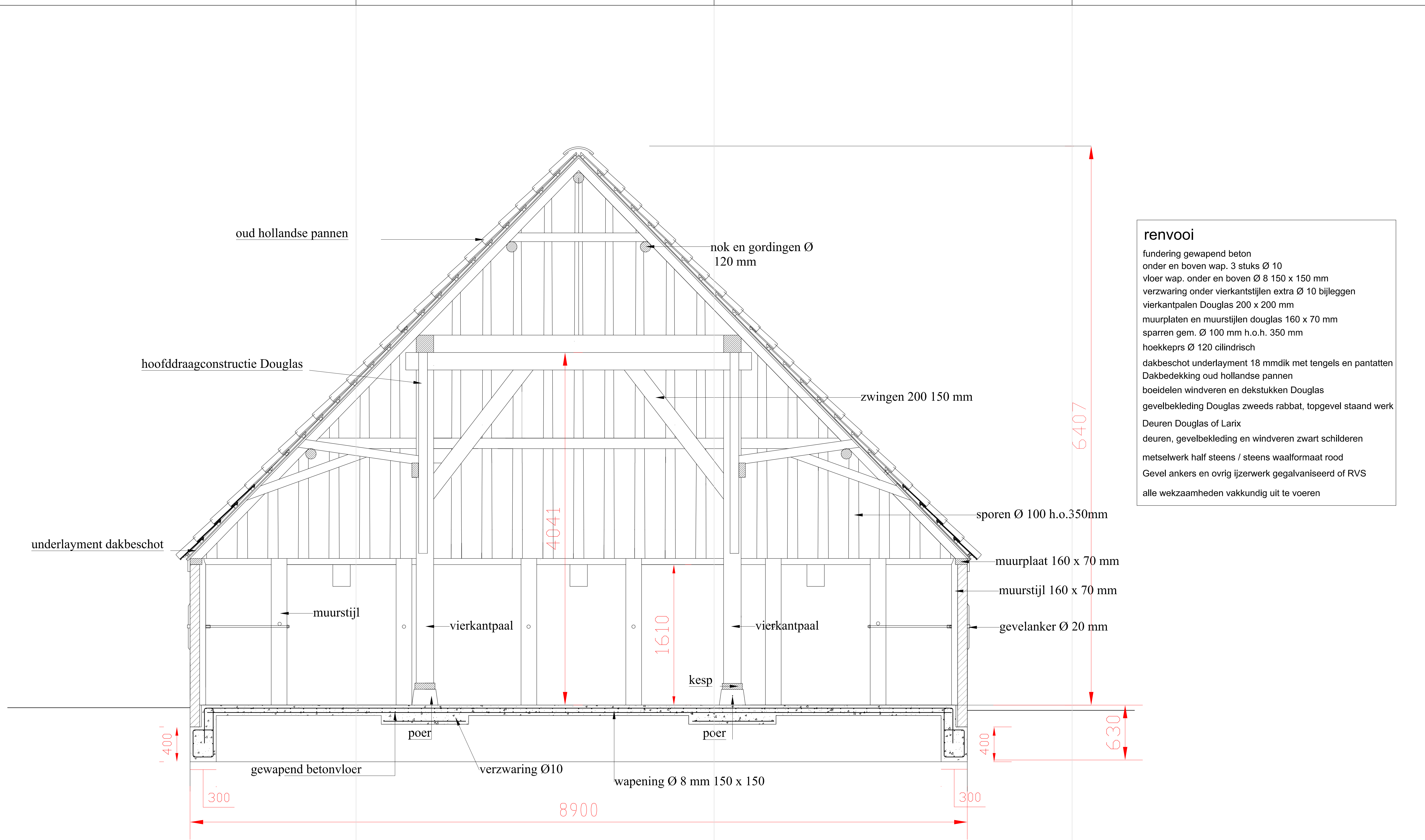
Doorsnede A-B
