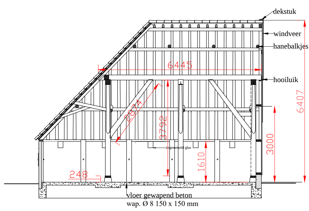
Doorsnede C-D
