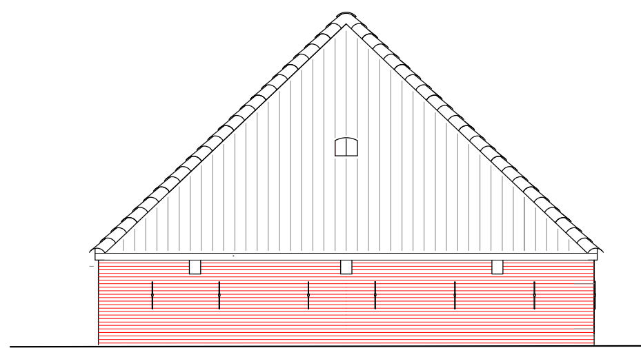
Achtergevel
