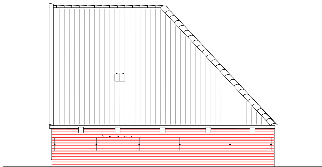
Rechter zijgevel
