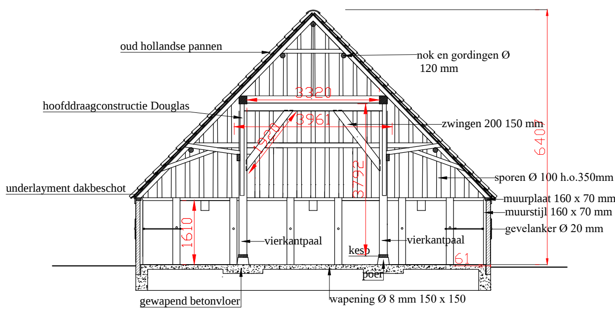
Doorsnede A-B
