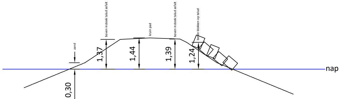
Profiel AA
