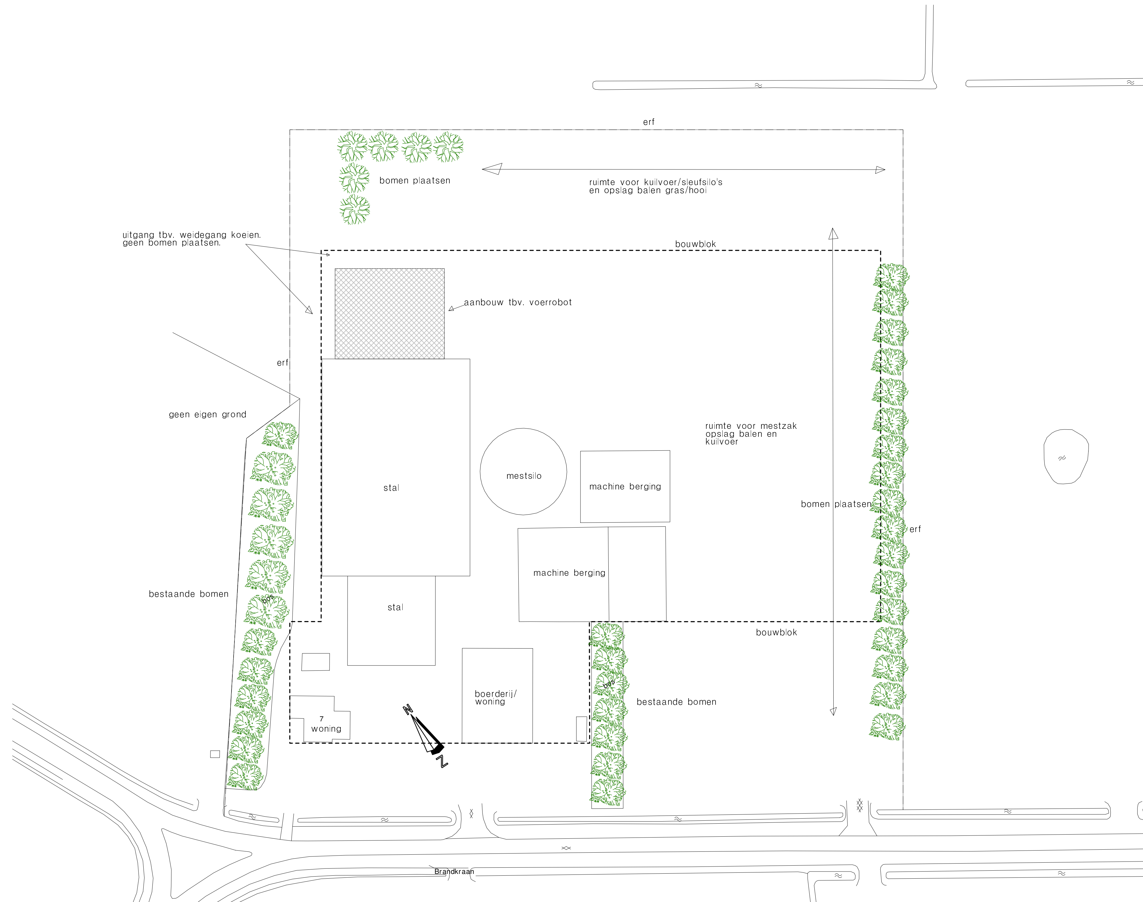
Erf inrichting tbv. vergroten stal met voerrobot ruimte. Situatie Oostkaap 7-9 te Oosterend Texel Schaal 1:500
