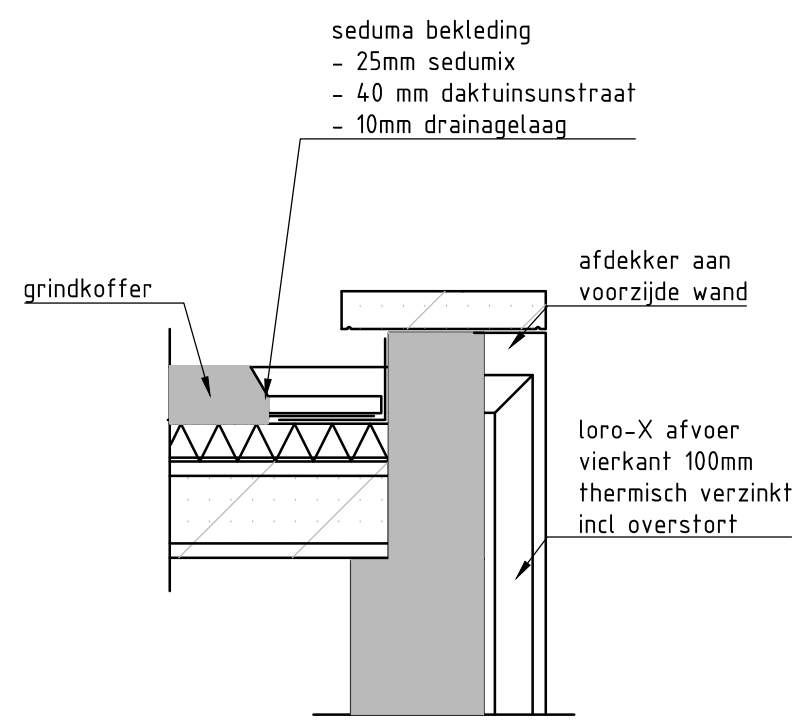
DETAIL 2: AFVOER schaal 1:20
