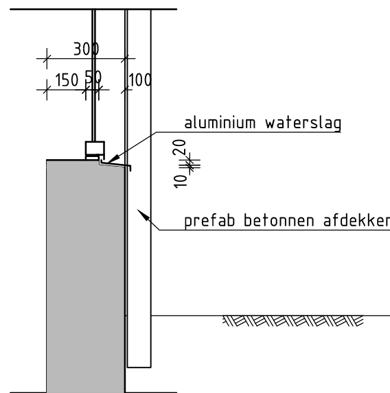
DETAIL 5: KOZIJN schaal 1:20
