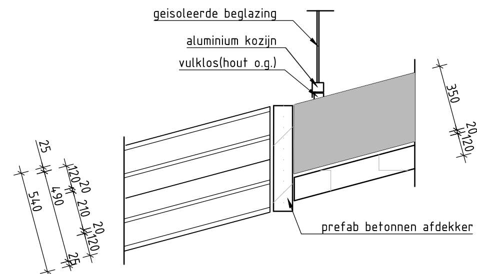
DETAIL 7: KOZIJN schaal 1:20
