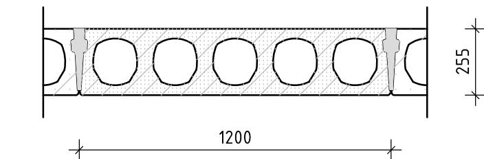
DOORSNEDE KANAALPLAAT K260/5 schaal 1:20
