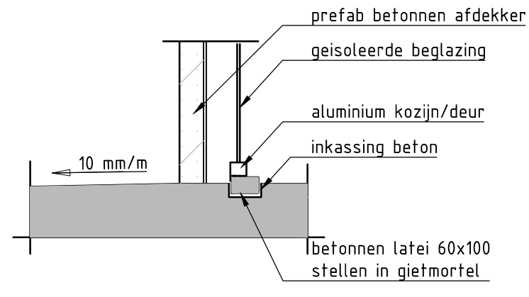
DETAIL 6: KOZIJN schaal 1:20
