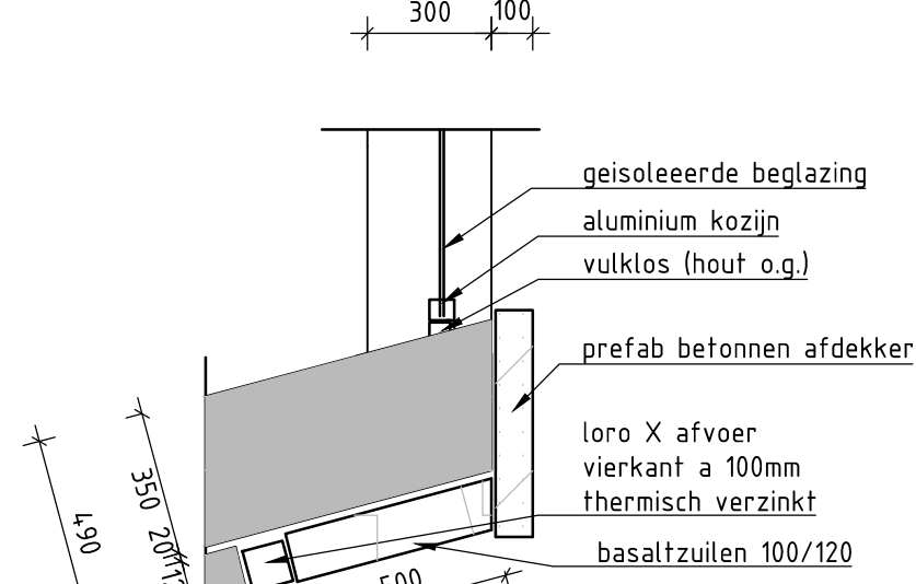
DETAIL 3: AFVOER schaal 1:20
