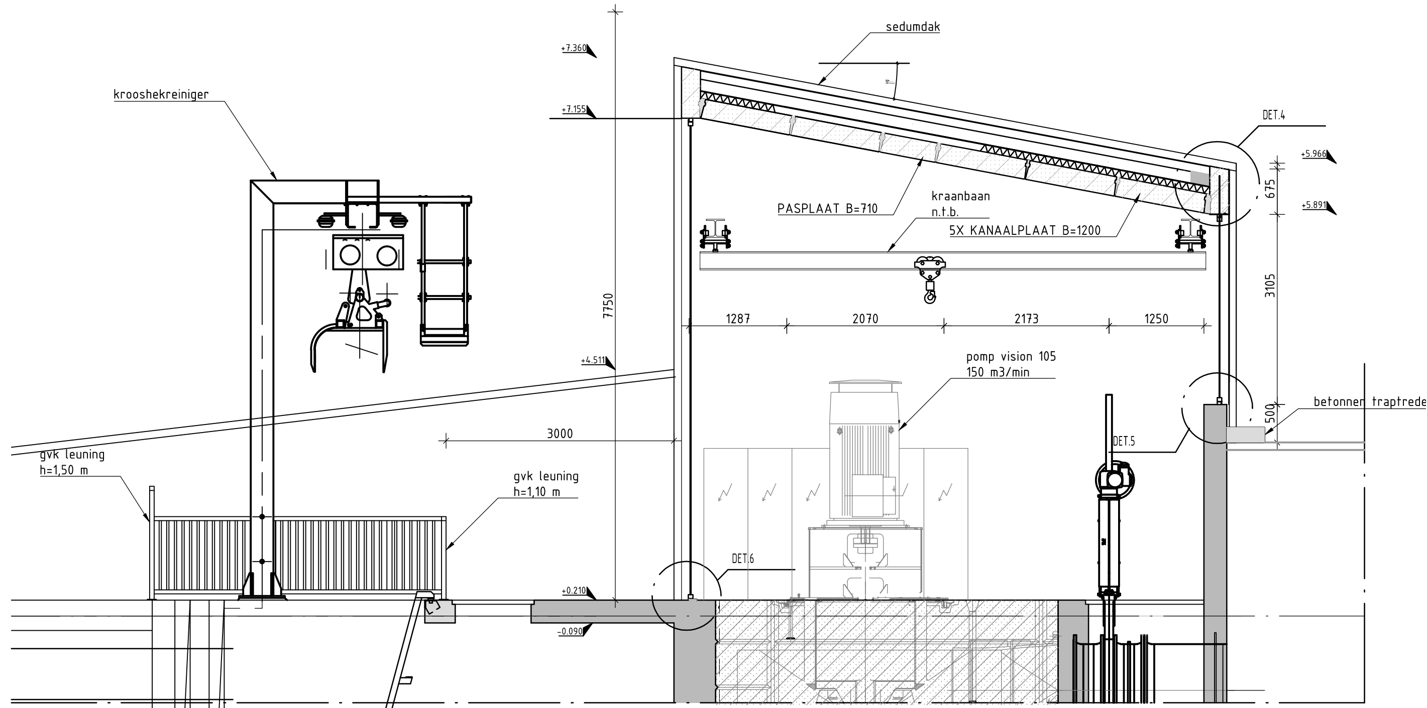
DOORSNEDE BOVENBOUW schaal 1:50
