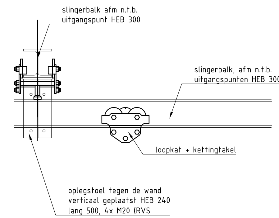
PRINCIEPEDETAIL HIJSBALK schaal 1:20
