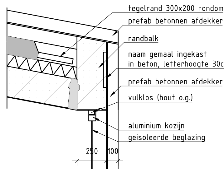
DETAIL 4: KOZIJN schaal 1:20
