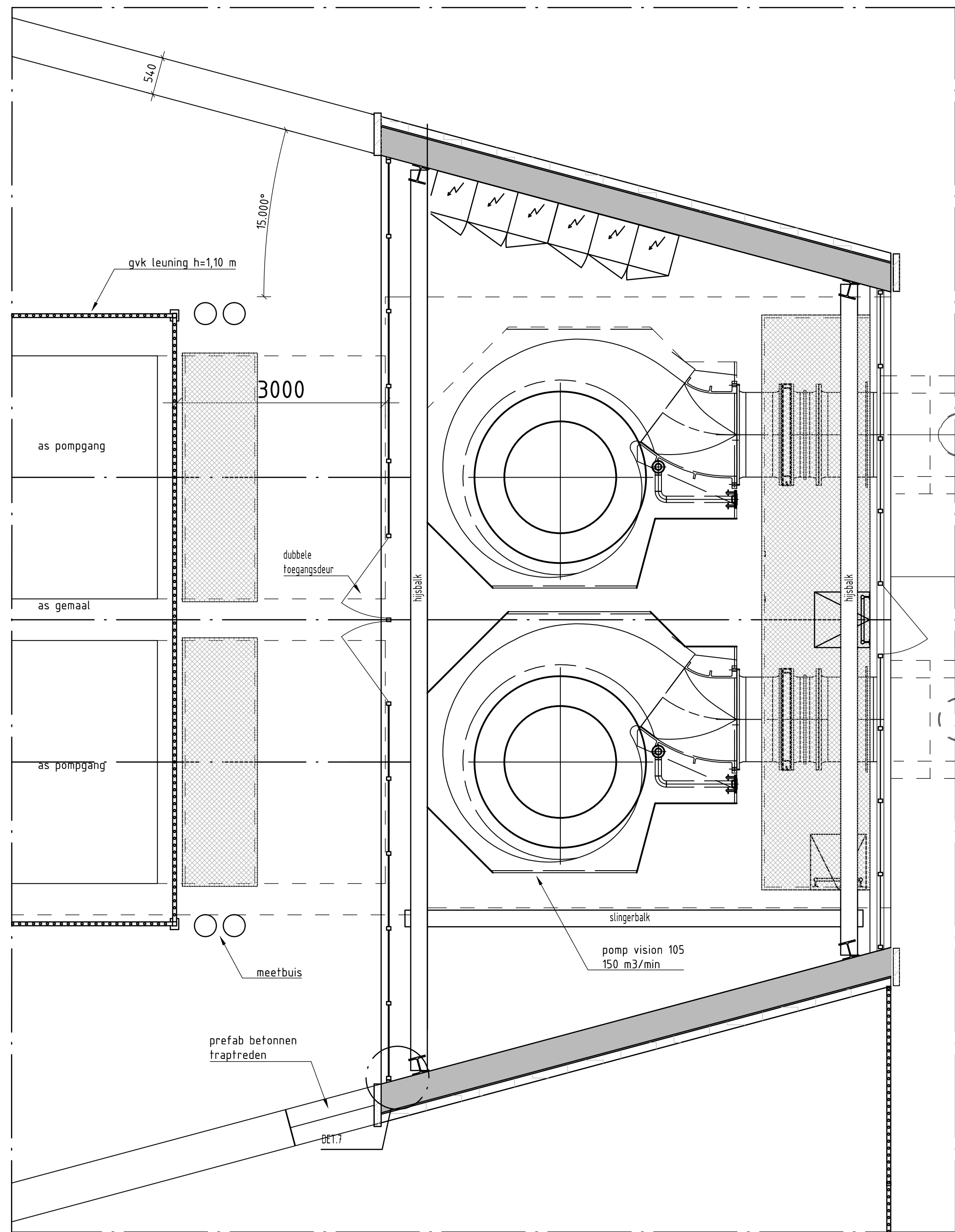
DOORSNEDE BOVENBOUW schaal 1:50
