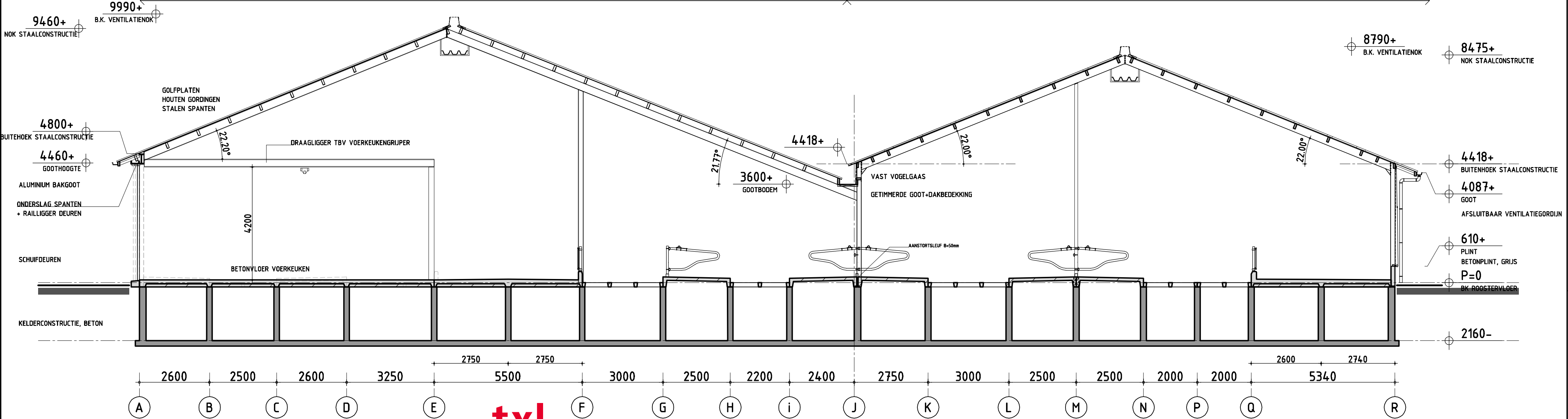
DOORSNEDE A-A
