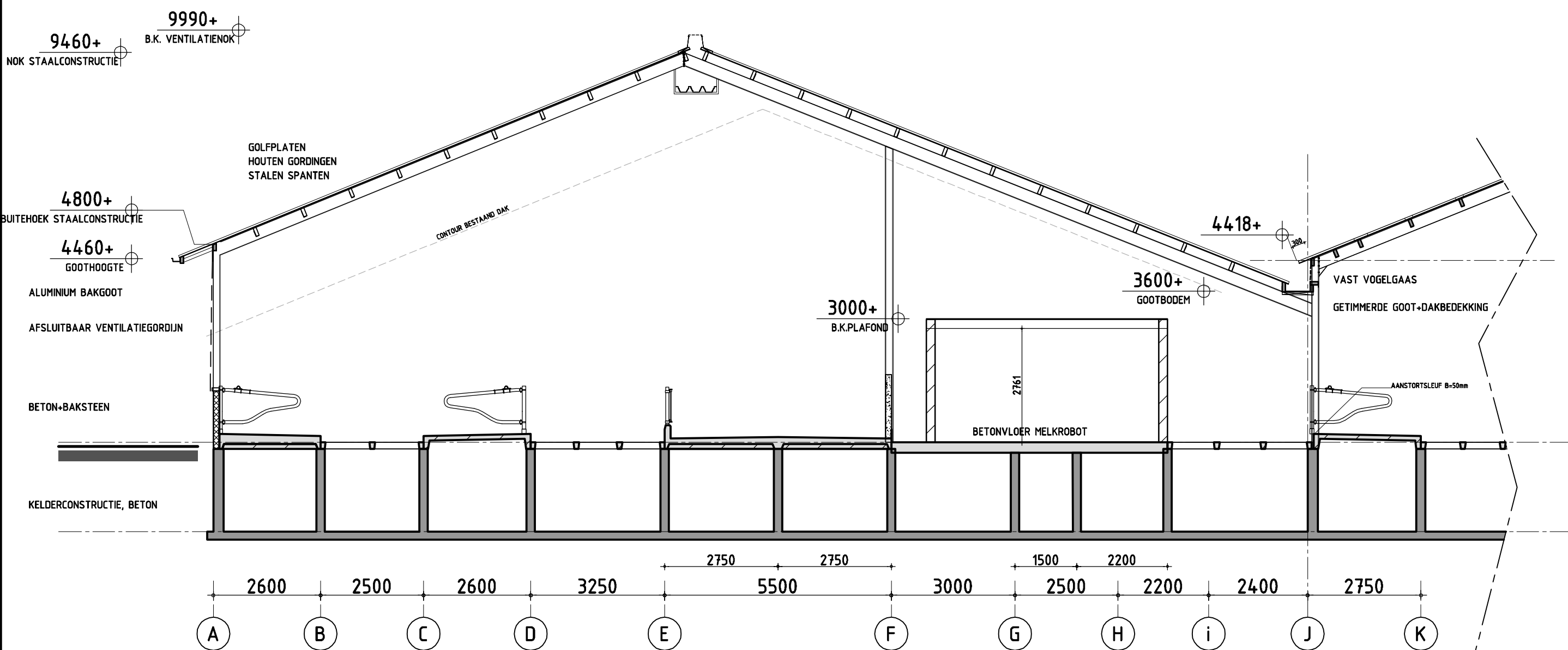
DOORSNEDE B-B
