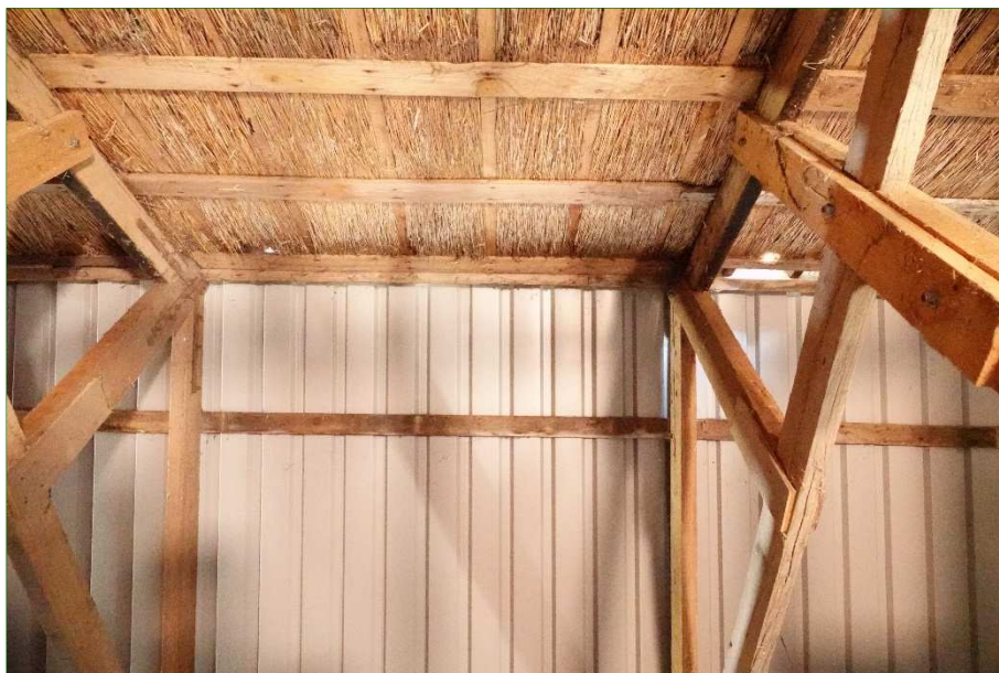
Dakbedekking van stalen sandwichplaten enerzijds en Riet onder dakpannen anderzijds.
