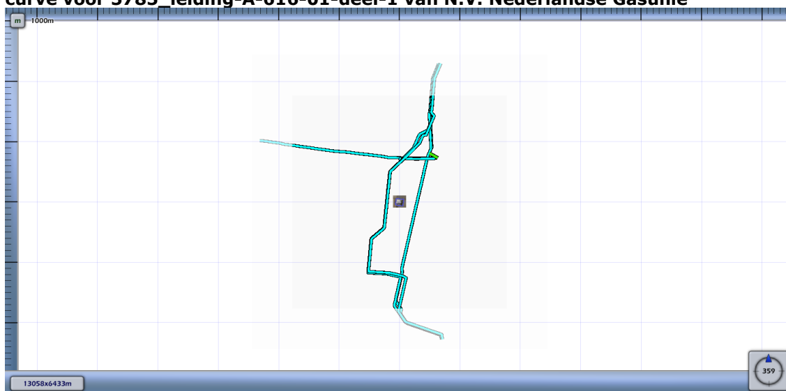
Figuur 4.4 Kilometer leiding behorende bij de maximale overschrijding van de FN-curve voor 5785_leiding-A-616-01-deel-1 van N.V. Nederlandse Gasunie
