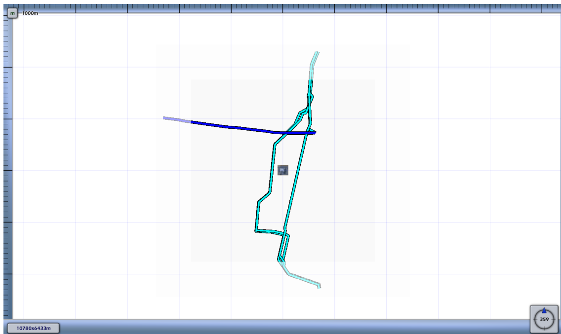
3.6 Figuur 3.6 Plaatsgebonden risico voor 5785_leiding-A-644-deel-1 van N.V. Nederlandse Gasunie
