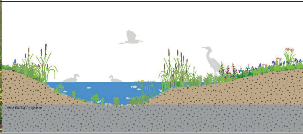
Doorsnede natuurvriendelijke oever
