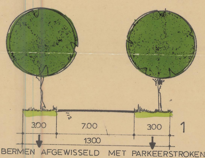
PRINCIPE PROFIEL SCHAAL 1:200
