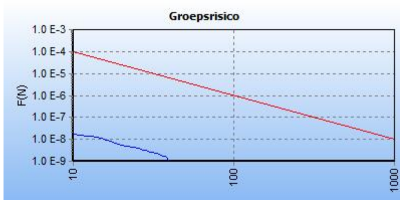
5.1 Figuur 5.1 FN curve voor 7235_leiding-A-637-deel-1 van N.V. Nederlandse Gasunie voor de kilometer tussen stationing 2070.00 en stationing 3070.00
