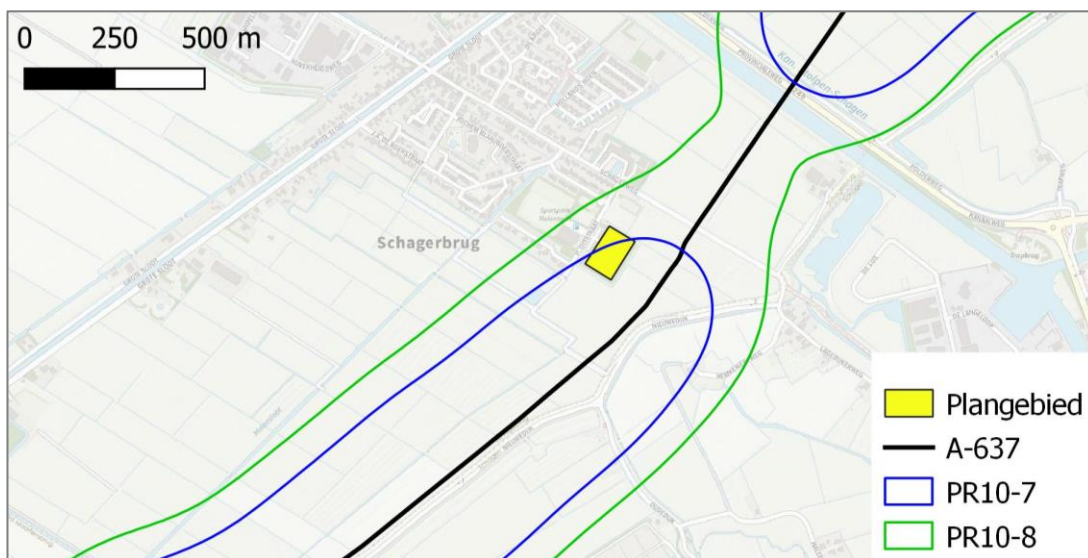
Figuur 3. PR-contouren aardgasleiding A-637
