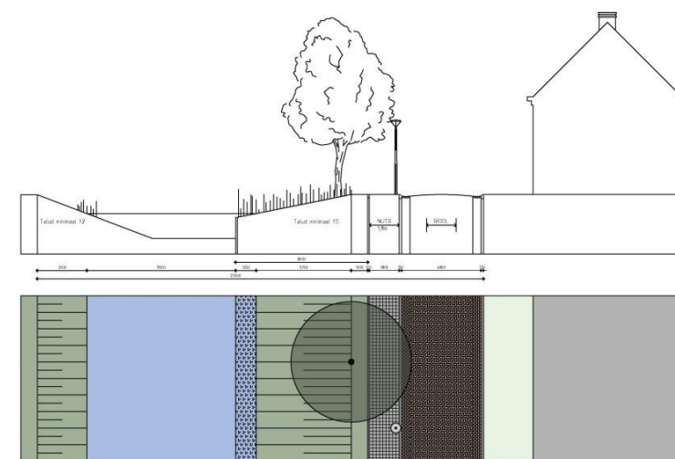
PROFIEL C-C
