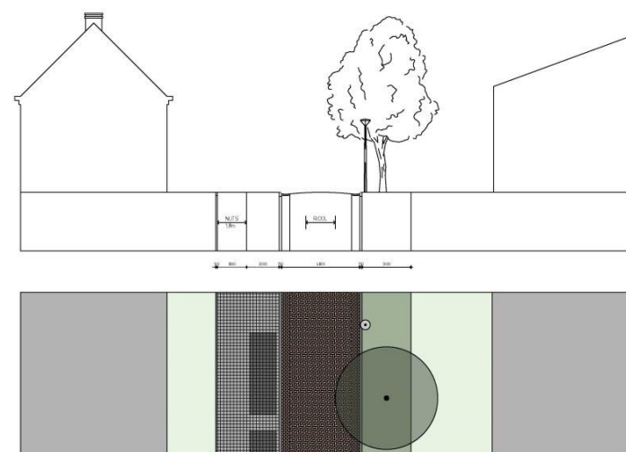
PROFIEL D-D
