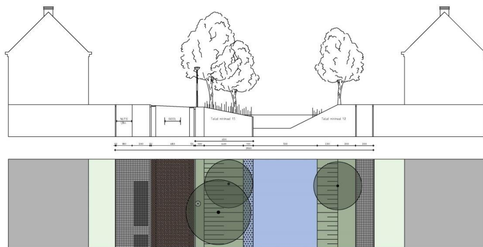
PROFIEL A-A
