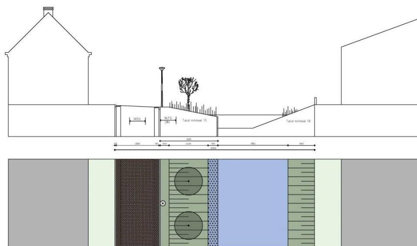
PROFIEL B-B
