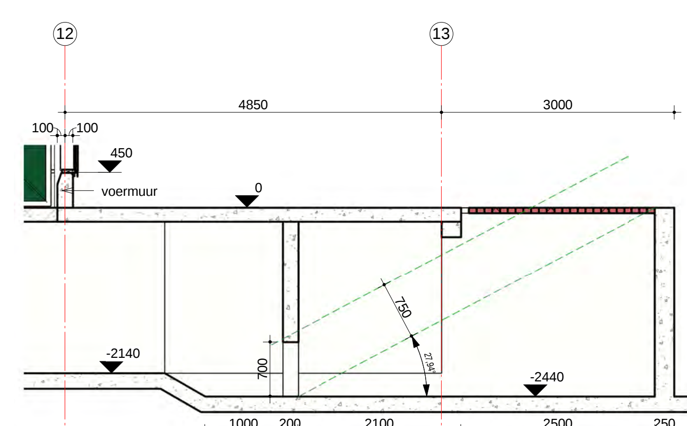
mixput 1 : 50
