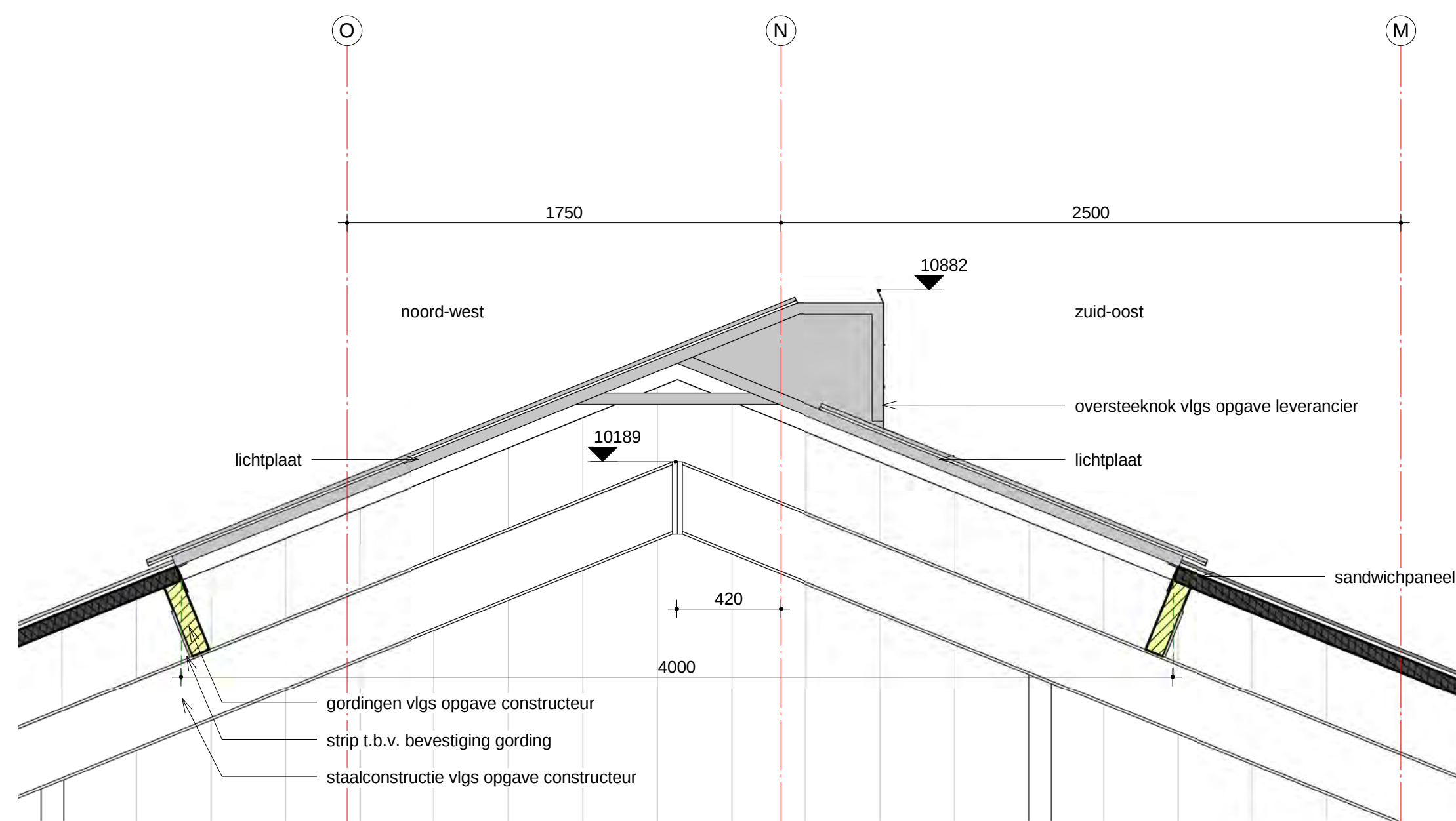
Det.2 1 : 20
