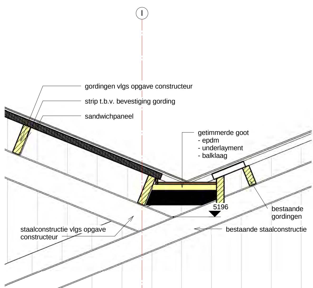
Det.3 1 : 20
