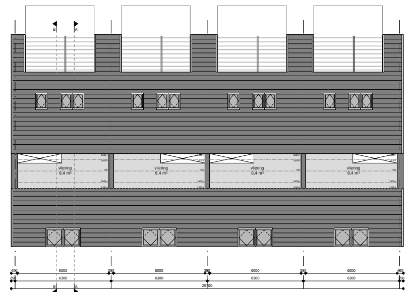
Vliering
