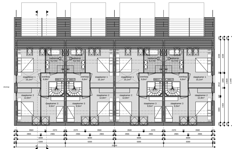
Tweede verdieping
