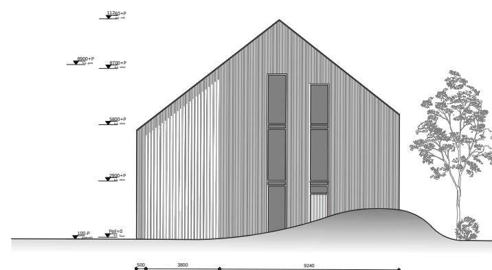
Rechter zijgevel
