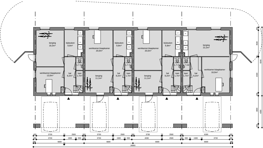
Begane grond
