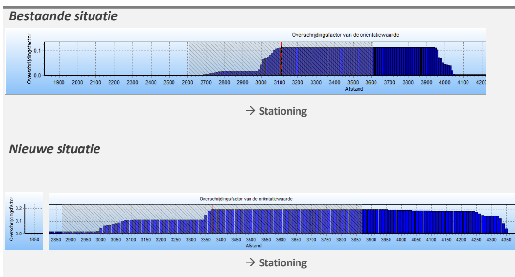
Figuur 6.3 Groepsrisico screening voor W-570-01 van Gasunie bestaand en nieuw
