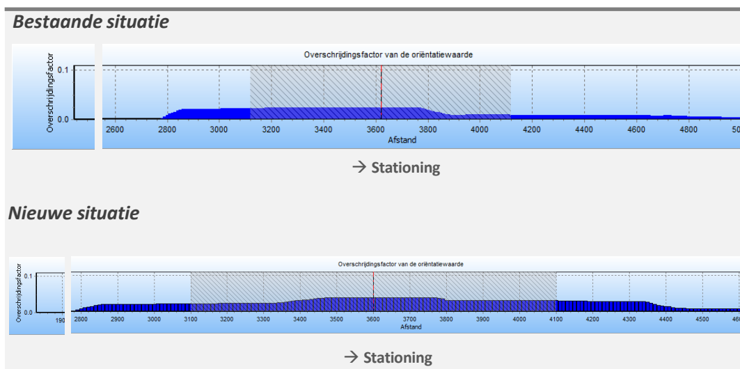
Figuur 6.5 Groepsrisico screening voor W-570-23 van Gasunie bestaand en nieuw
