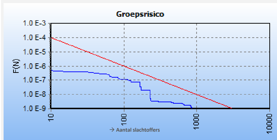
Figuur 6.4 FN curve voor buisleiding W-570-01 van Gasunie voor de kilometer tussen stationing 2610.00 en 3610.00 (bestaande situatie) en stationing 2870.00 en 3870.00(nieuwe situatie)
