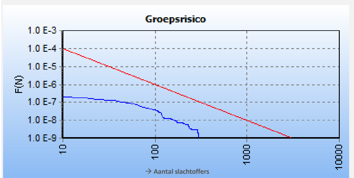
Figuur 6.6 FN curve voor buisleiding W-570-23 van Gasunie voor de kilometer tussen stationing 3120.00 en 4120.00 (bestaande situatie) en 3100.00 en 4100.00 (nieuwe situatie)
