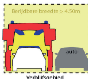
Figuur 4.8: Minimale berijdbare breedte van een tweerichtings-erftoegangsweg
