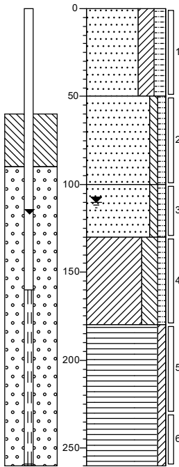
Boring: 01 Boormeester: Hans Manshanden
