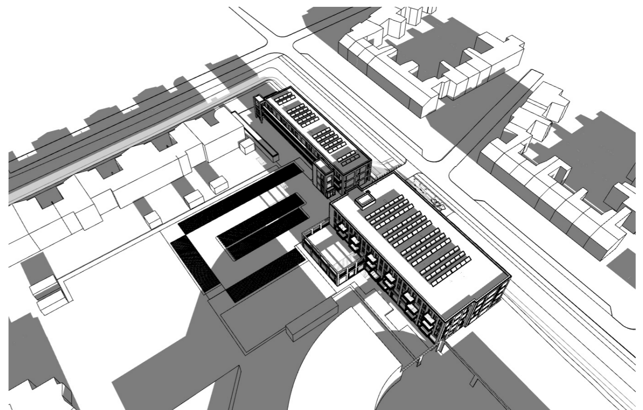
21 december / 12.00 uur / ZONDER BOMEN
