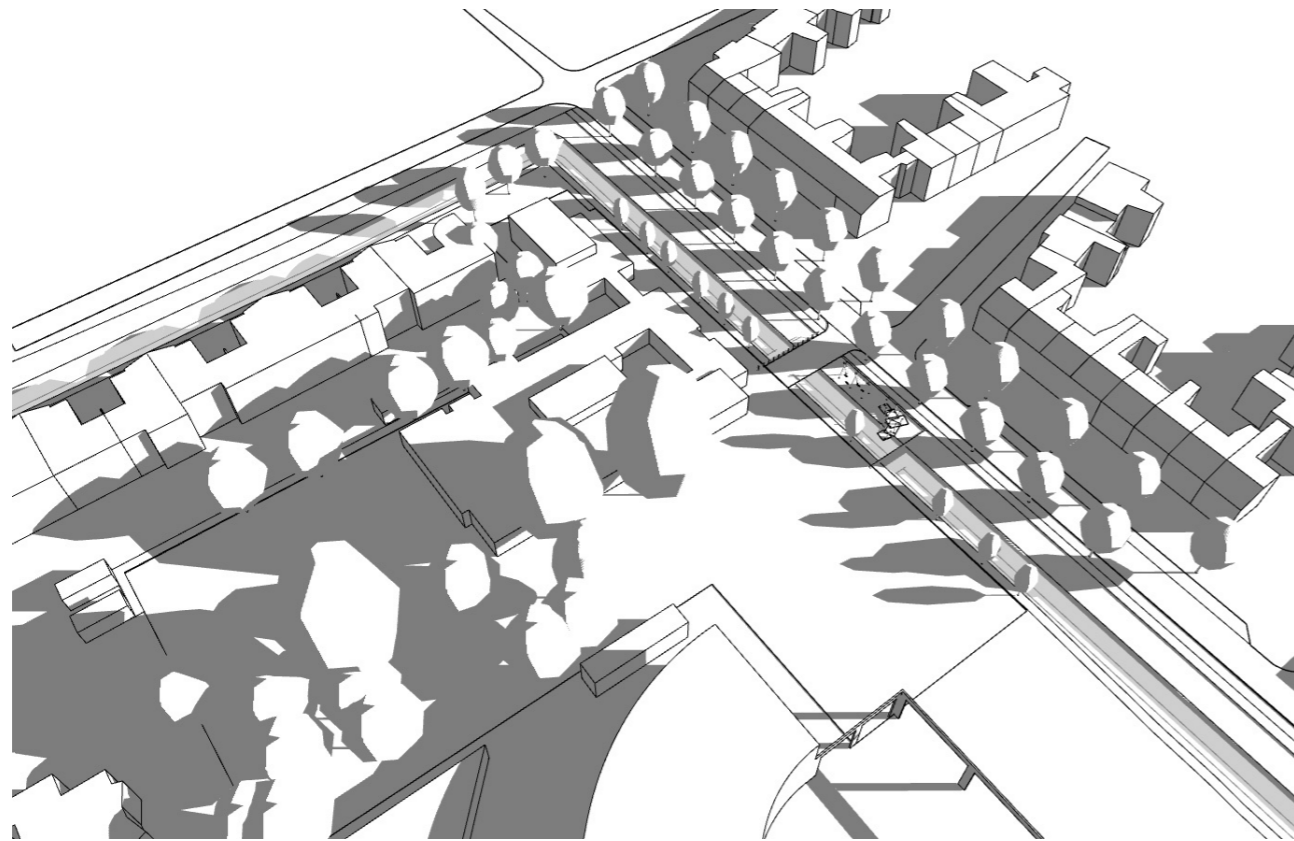
21 maart / 21 september / 9.00 uur / BESTAAND
