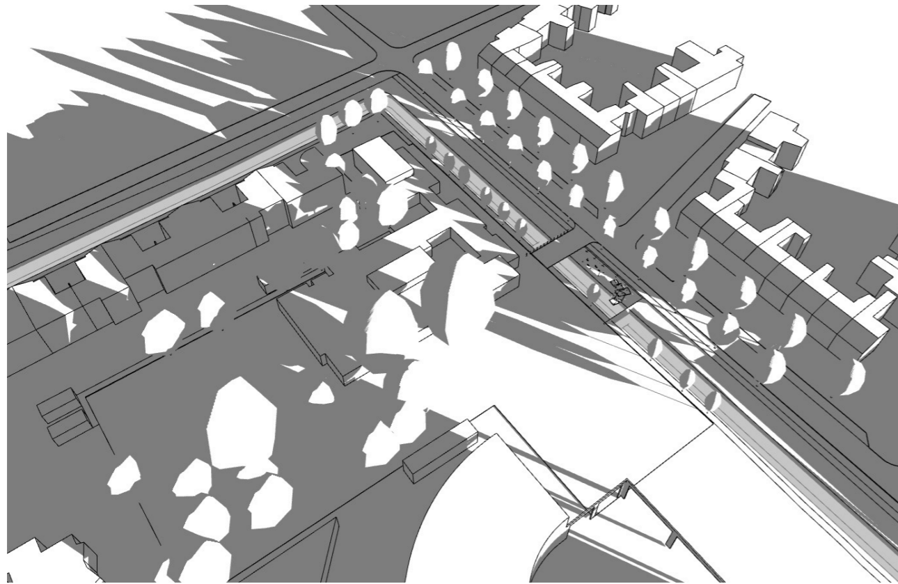
21 december / 10.00 uur / BESTAAND
