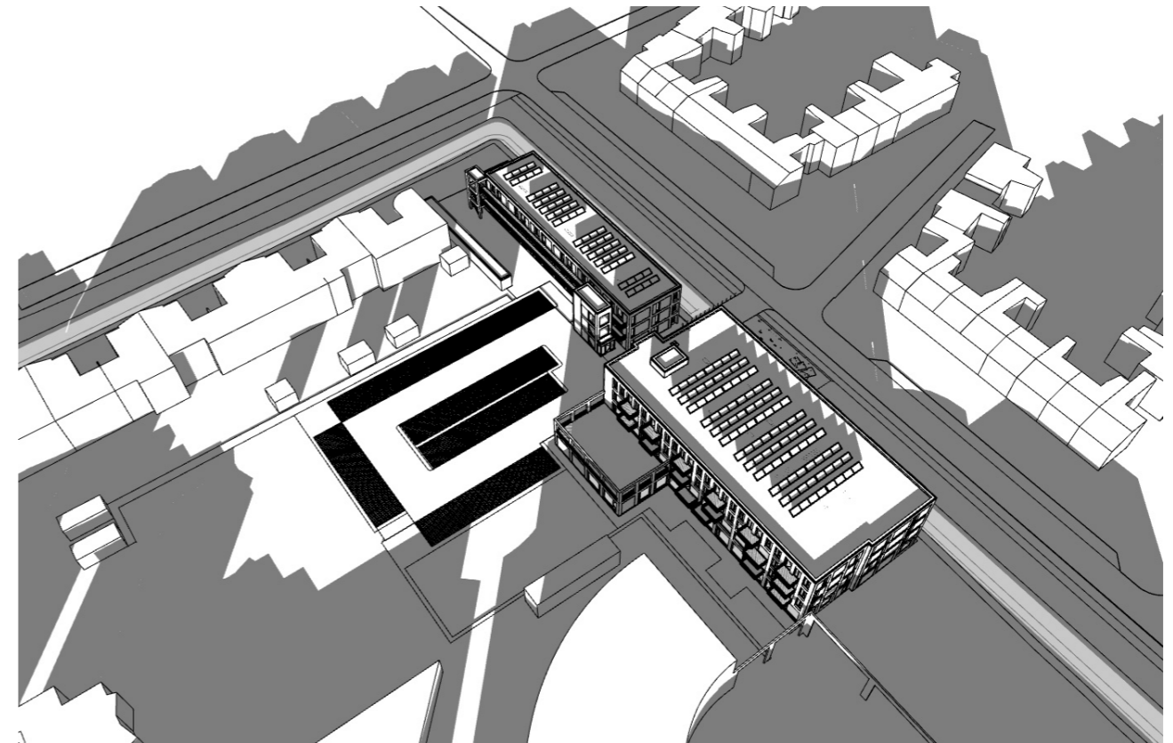
21 december / 15.00 uur / ZONDER BOMEN
