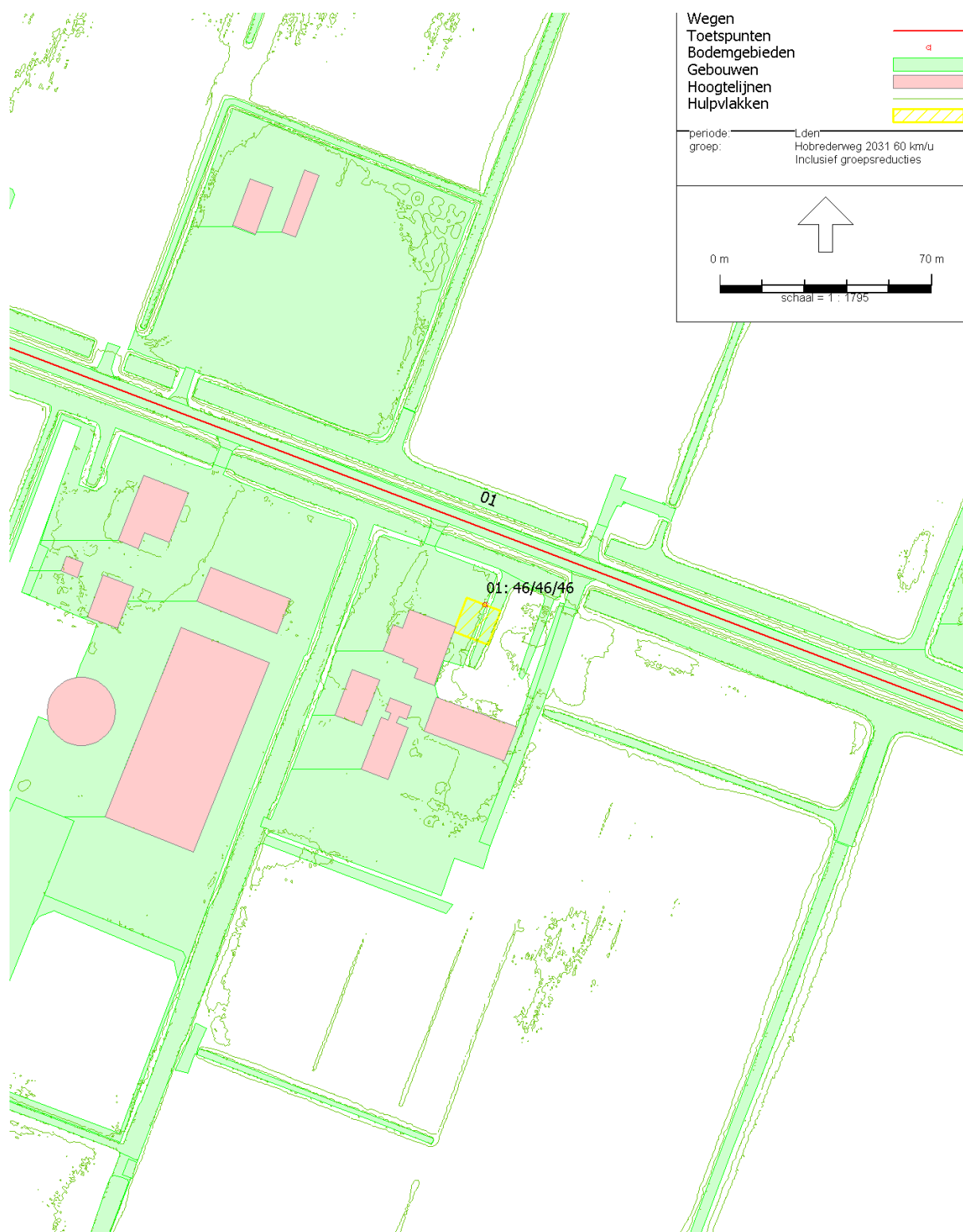
Figuur 5-1 Geluidbelasting Hobrederweg 2031 inclusief 5 dB aftrek artikel 110 Wgh
