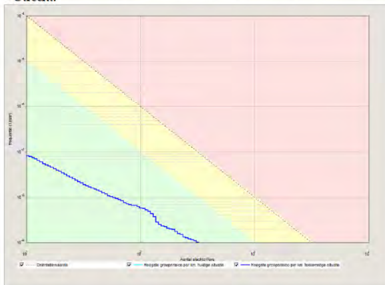
Abbeelding 8: fN-curves spoortraject Amsterdam - Utrecht huidige en toekomstige situatie.
