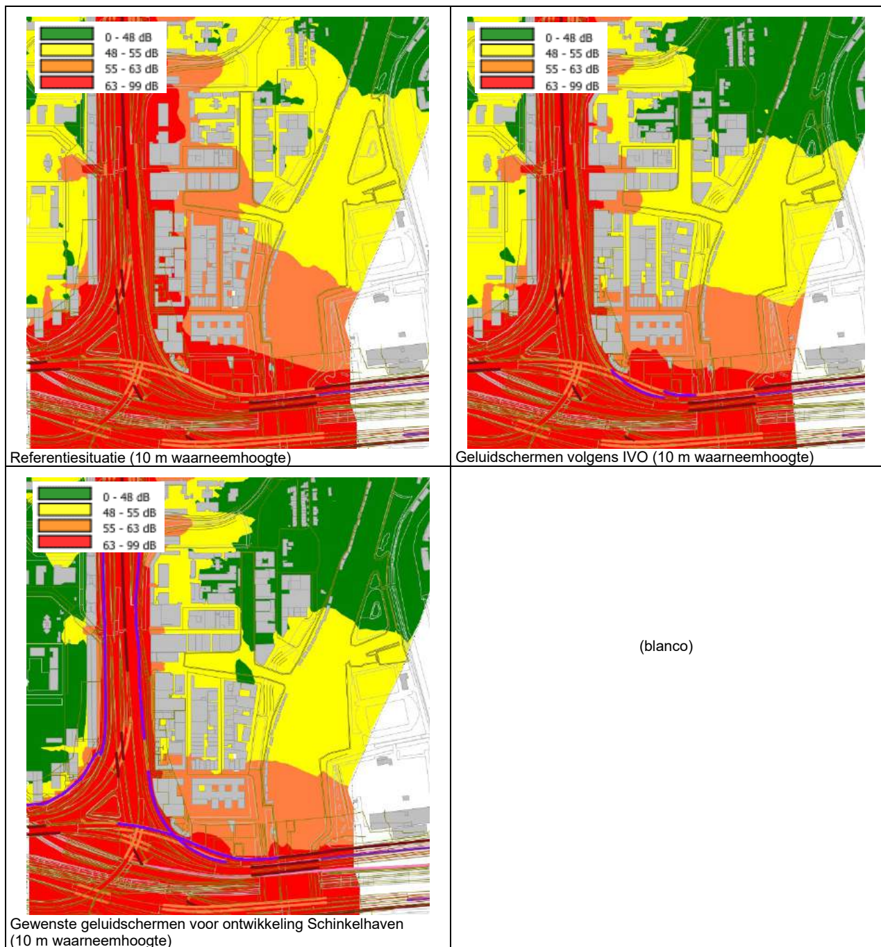
Figuur 6: Geluidscntouren snelweggeluid op waarneemhoogte 10 m
