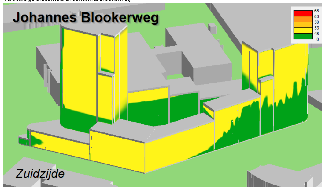
f5.2 Verticale geluidcontouren Johannes Blookerweg
