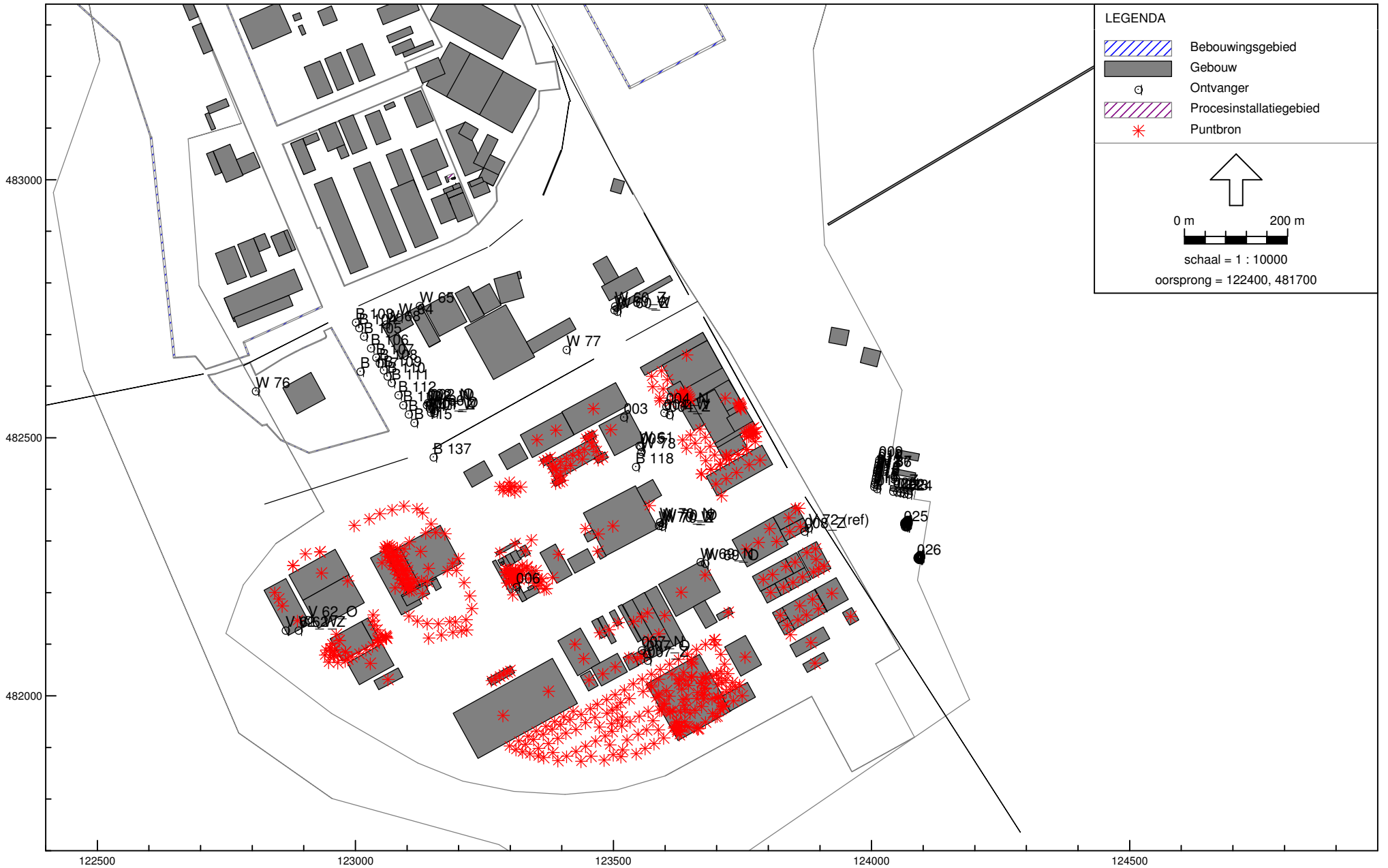
Overzicht rekenmodel
