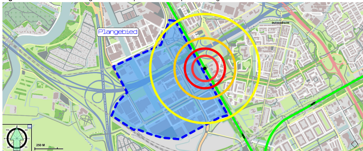
Figuur 4. Schematische weergave na een explosie van een spoorketelwagon LPG
