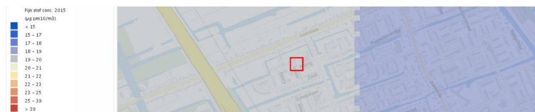
Abbeelding 7: Concentratie PM 10 in het jaar 2015.
