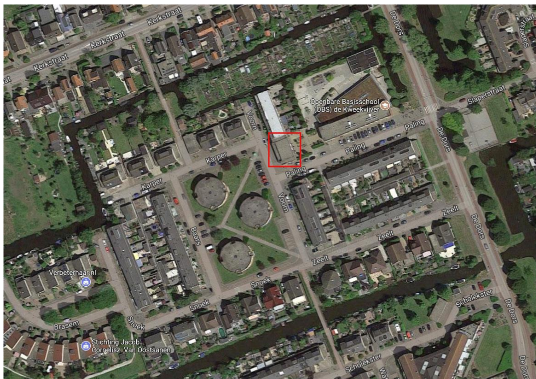
Afbeelding 1: Ligging plangebied.
