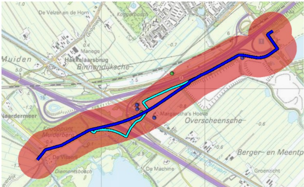
Figuur 2 Bevolkingsgegevens rondom de W-533-19 zoals aangeleverd door Bridgis. Groen gekleurde punten zijn adressen met als hoofdfunctie wonen en blauw gekleurde punten zijn adressen met als hoofdfunctie werken of gemengd. Het invloedsgebied van de leiding (na verlegging) is weergegeven in het rood.
