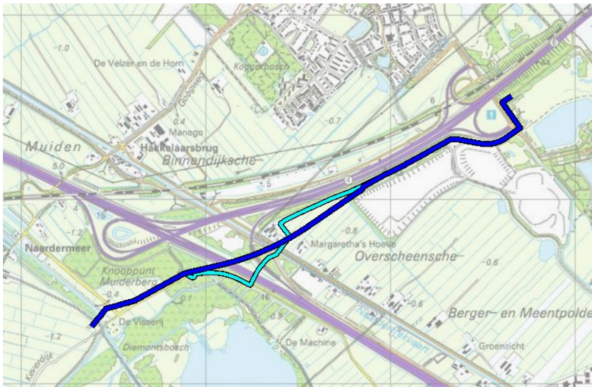
Figuur 1 Ligging van de leiding W-533-19 op een topografische kaart. De ligging van de leiding na verlegging is weergegeven in het donkerblauw; de ligging van de leiding voor verlegging is weergegeven in het lichtblauw.
