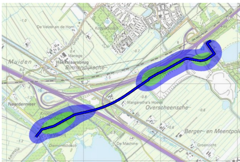
Figuur 3 Ligging van gastransportleiding W-533-19 (blauw) in de toekomstige situatie. De contouren van het PR van 10^{-7} en 10^{-8} per jaar van de leiding worden respectievelijk weergegeven met groene en blauwe gebieden.
