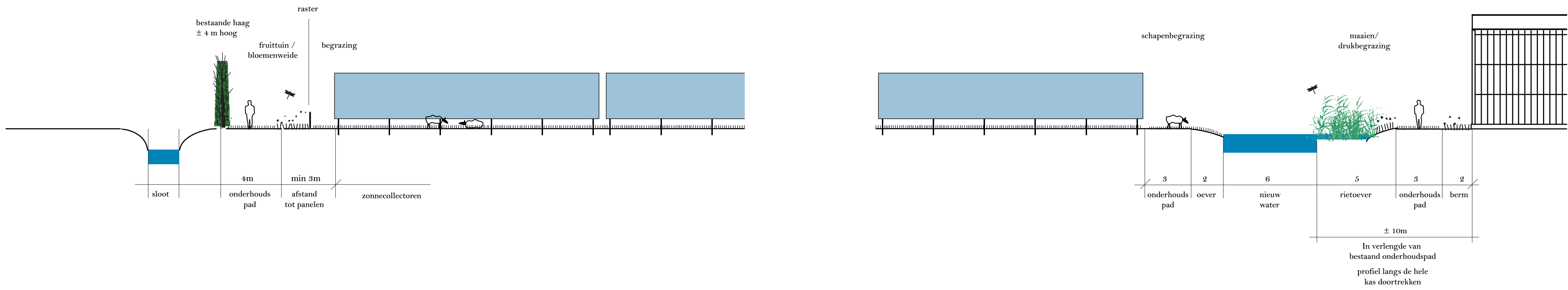
Profiel E
