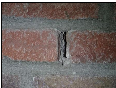
Figuur 13. Open stootvoeg die toegang geeft tot de spouwmuur.
