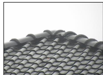
Figuur 12. Aanwezig ondervorstband onder de nokpannen.
