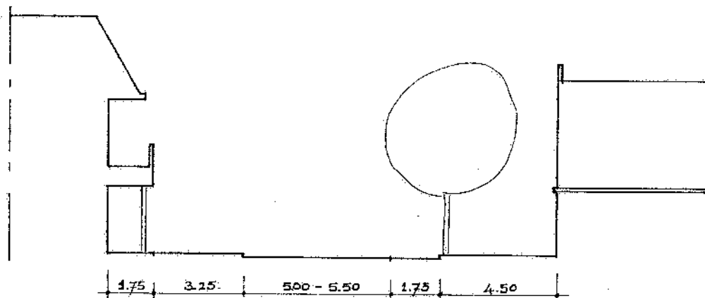
PROFIEL 5-5
