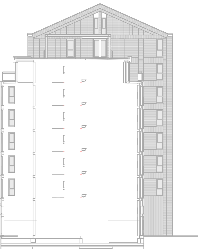
Rechter Zijgevel pakhuis
