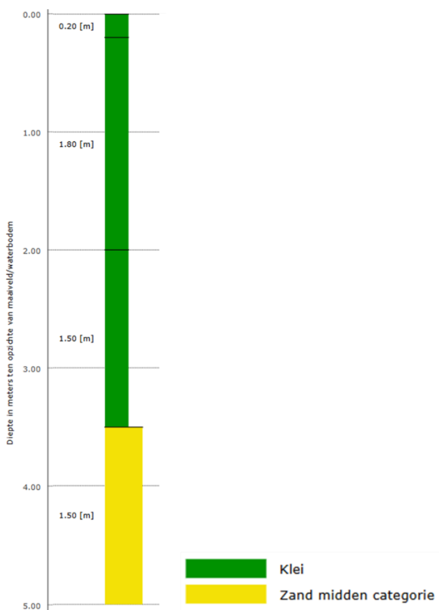
Figuur 4.2 Boorprofiel B19F0601
