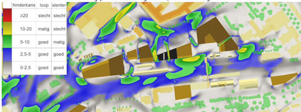
f3.2 Het te verwachten windklimaat in de geplande bebouwingssituatie, beoordeeld volgens de NEN 8100
