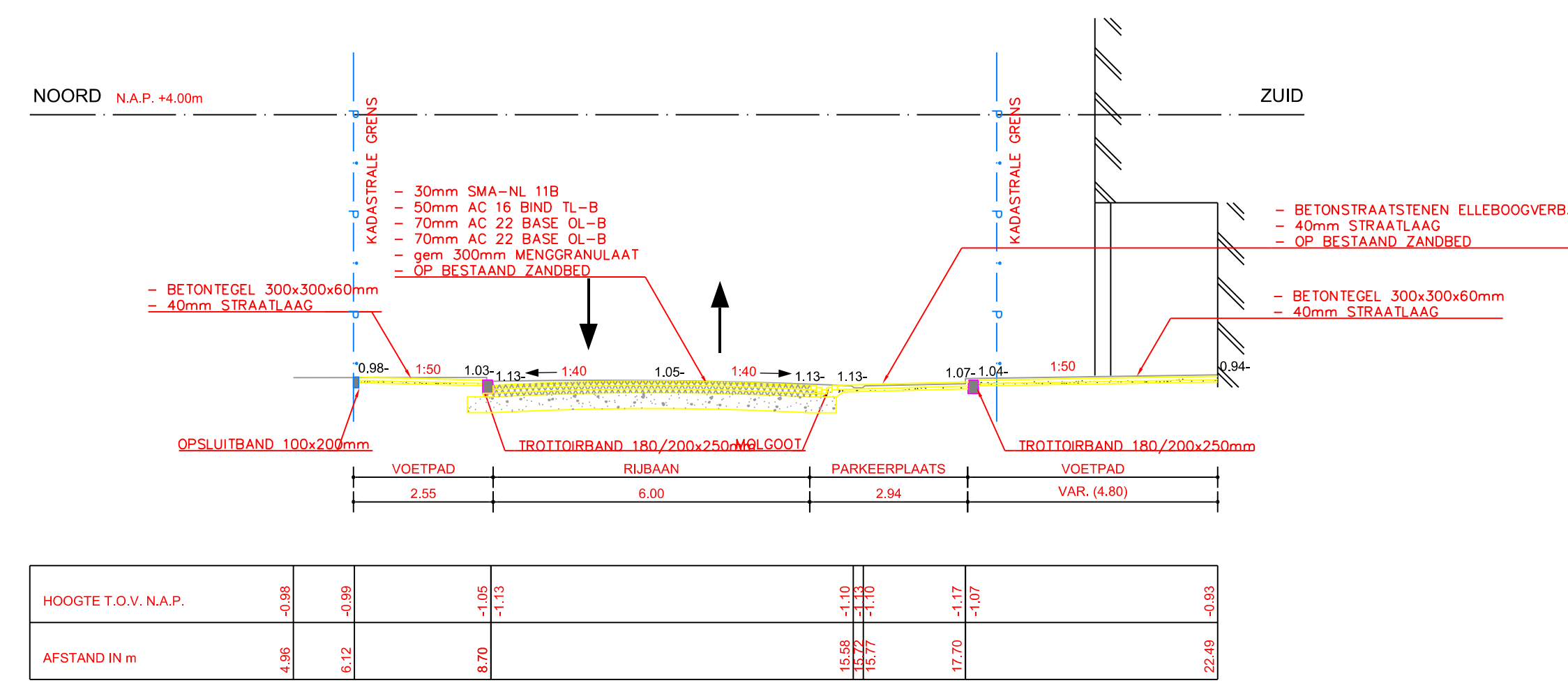
DWARSPROFIEL 6 SCHAAL 1:100
