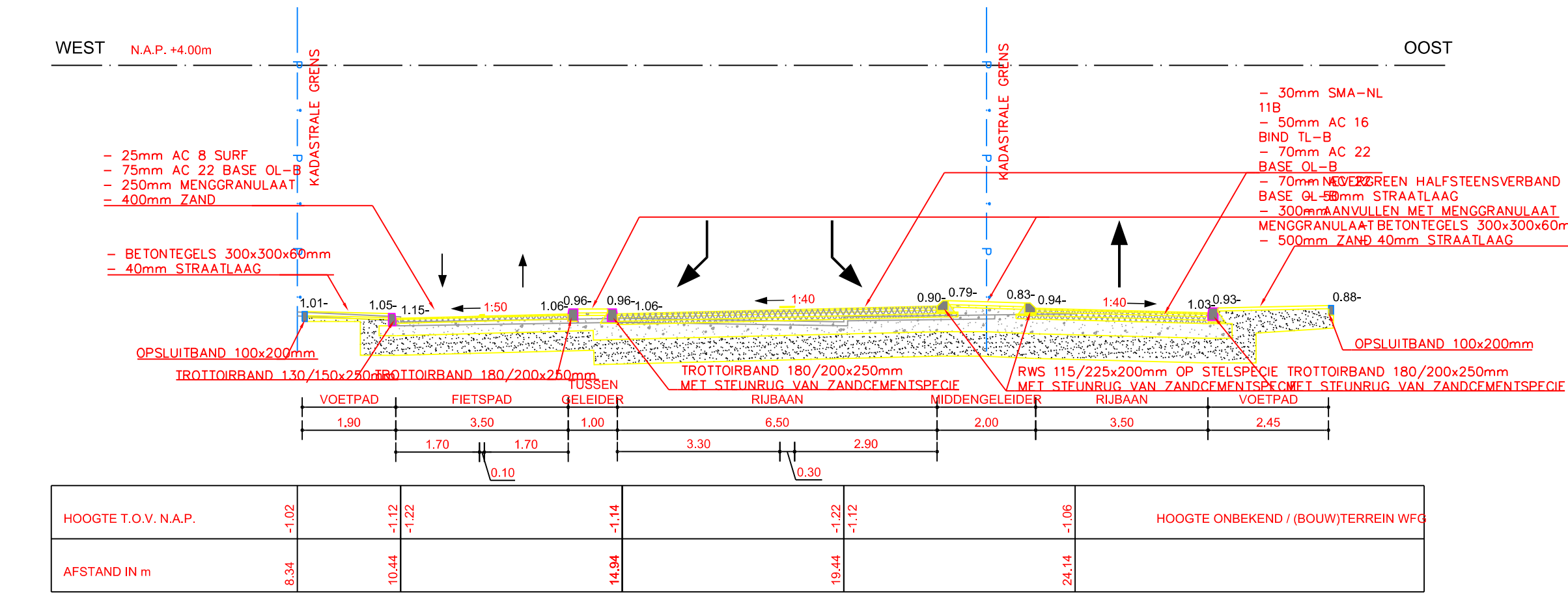
DWARSPROFIEL 9 SCHAAL 1:100
