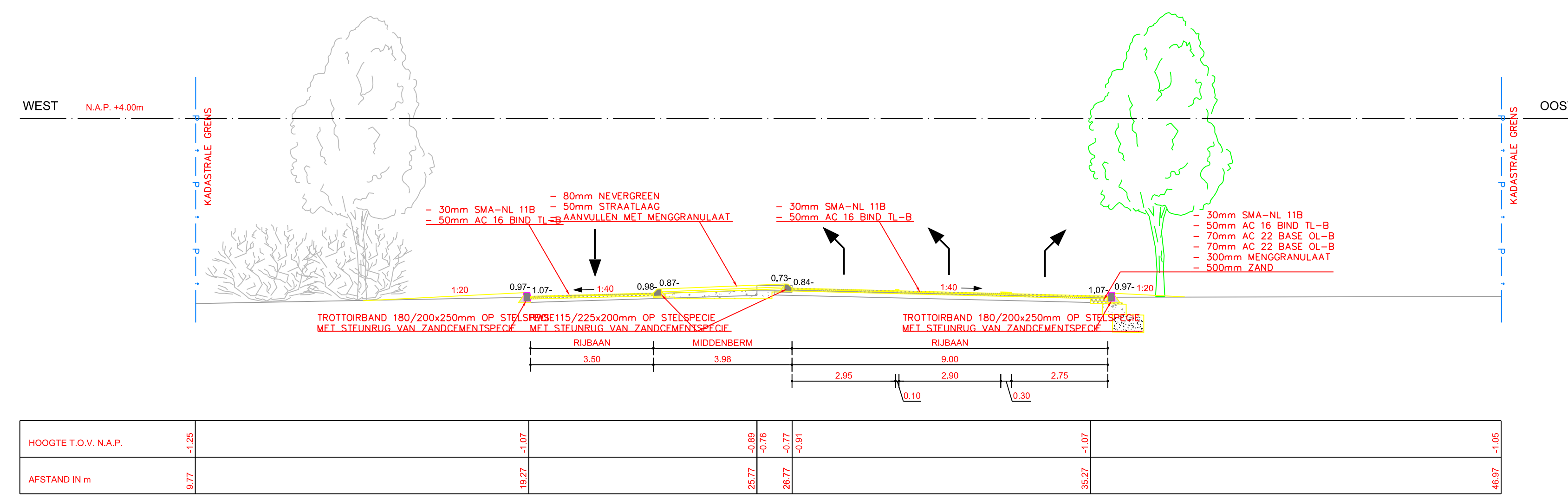
DWARSPROFIEL 5 SCHAAL 1:100
