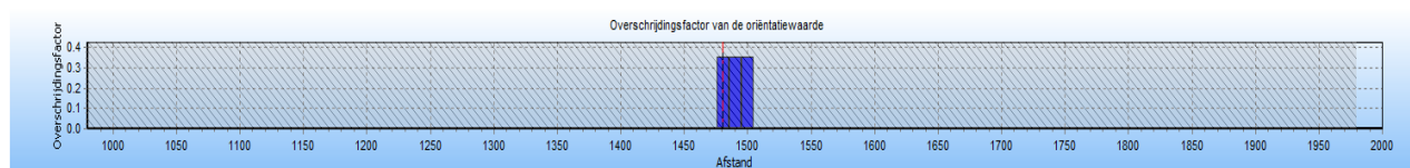
Figuur 5 Overschrijding van het groepsrisico als functie van de stationing van de W-500-19.
