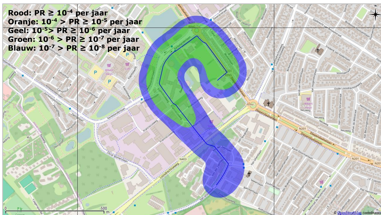
Figuur 4 PR van gastransportleiding W-500-19 (donkerblauw) in de toekomstige situatie.
