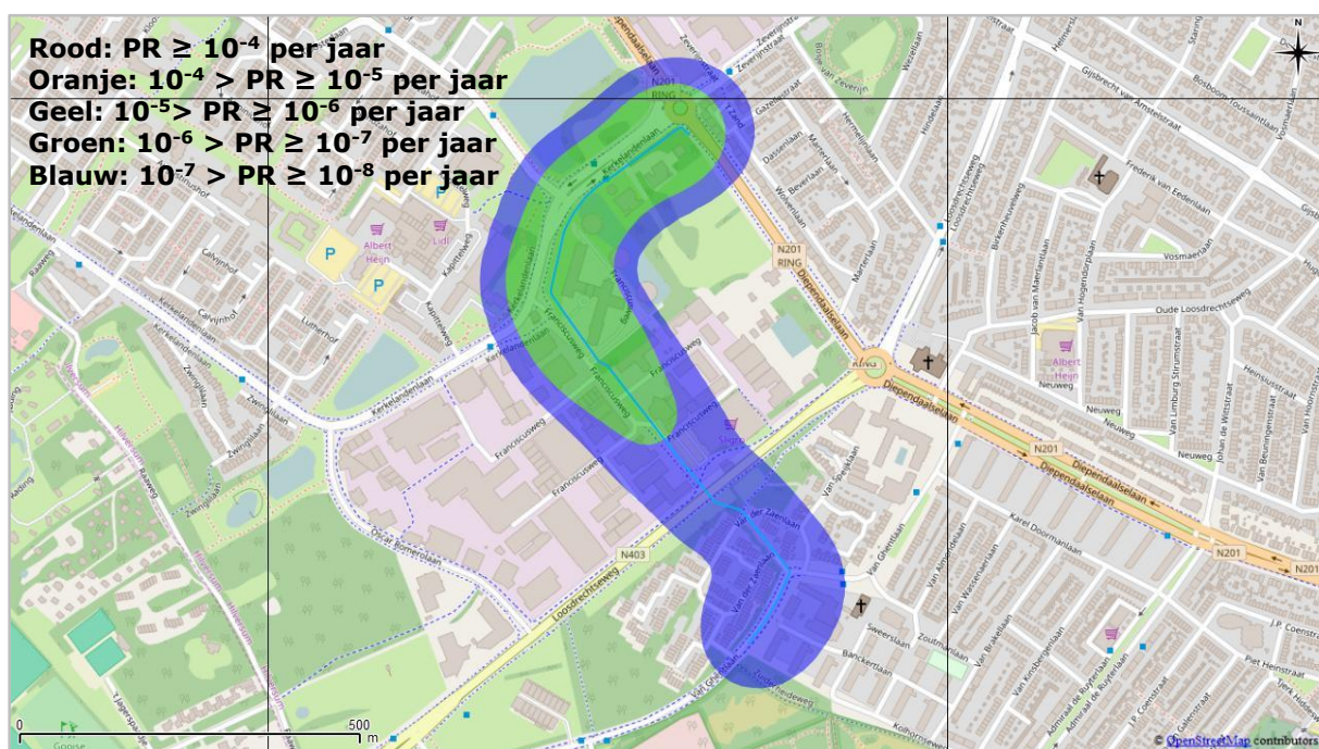
Figuur 3 PR van gastransportleiding W-500-19 (lichtblauw) in de huidige situatie.
