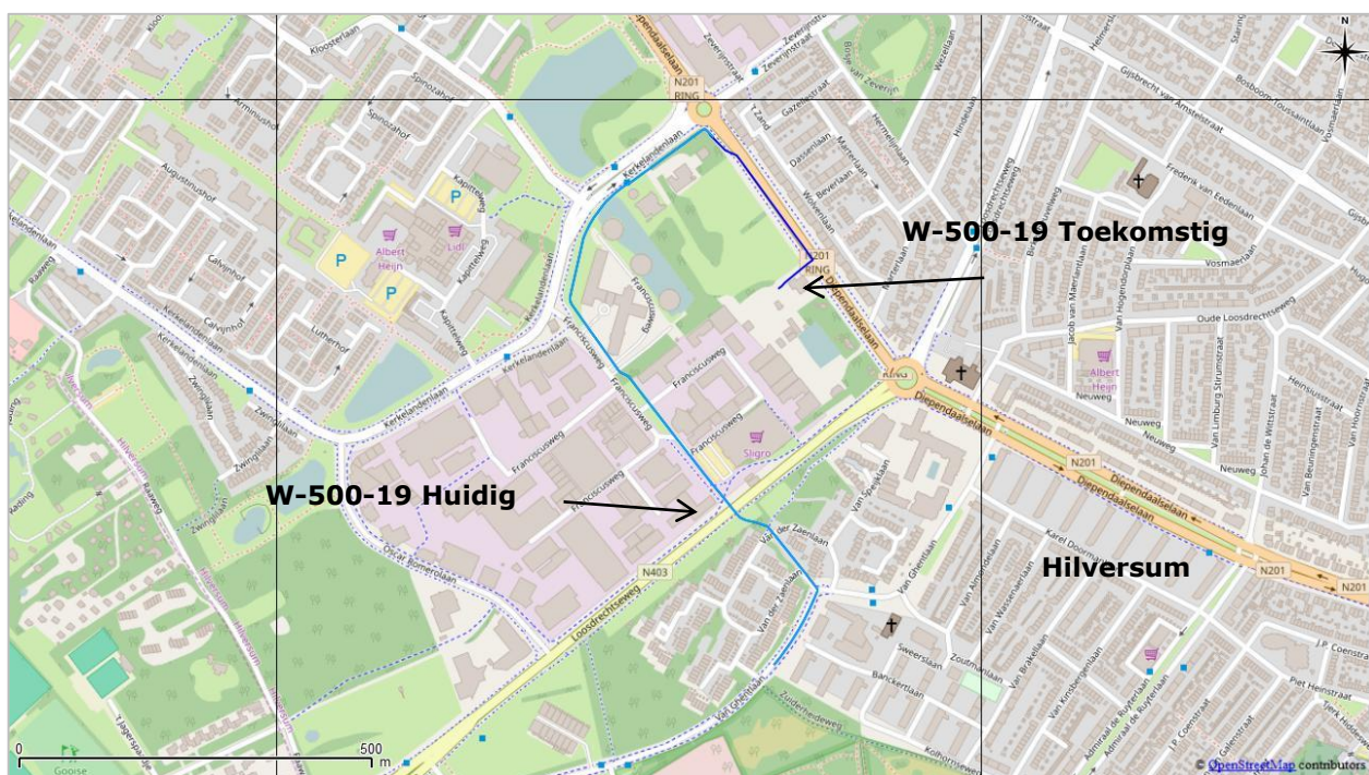
Figuur 1 Ligging van gastransportleiding W-500-19 in de huidige situatie (lichtblauw) en in de toekomstige situatie (donkerblauw).
