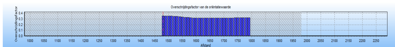
Figuur 8 Overschrijding van het groepsrisico als functie van de stationing van de W-500-19.
