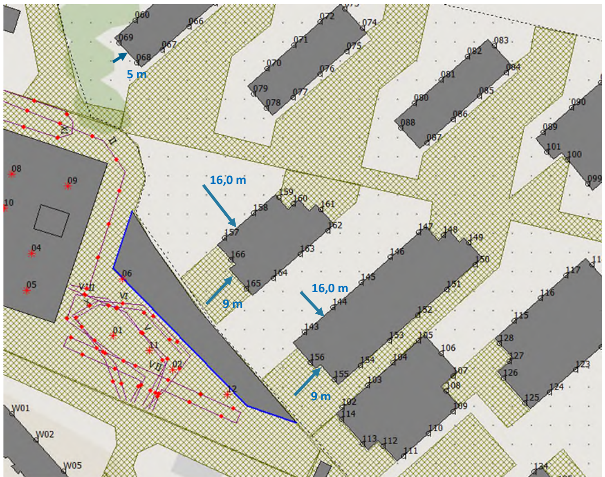
Afbeelding 5.2 Opschuiven appartementencomplex binnen stedenbouwkundig plan
