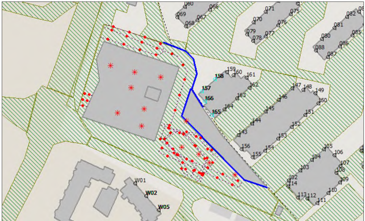
Afbeelding 5.1 Geluidscherm (hoogte 10,5 meter)
