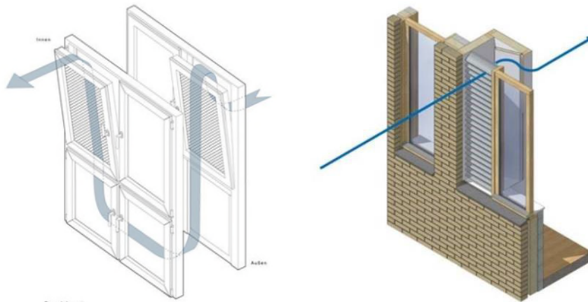
Afbeelding 5.6 Voorbeeld voorziening voor het creëren van een geluidluwe gevel met spui mogelijkheid
