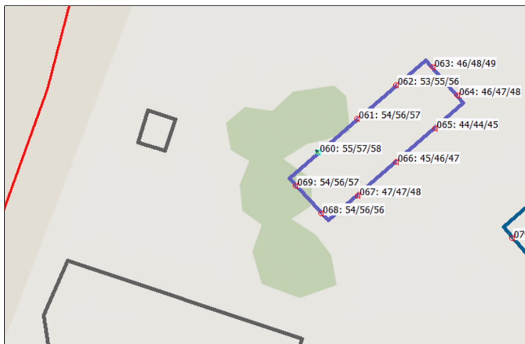
Afbeelding 4.2 Geluidbelasting ( L_{den} ) als gevolg van Kamerlingh Onnesweg, excl. aftrek ex artikel 110g Wgh (beoordelingshoogte 1,5 – 4,5 - 7,5 meter)
