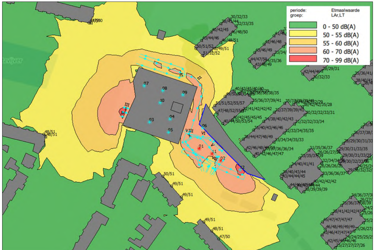
Afbeelding 4.4 Geluidcontour (etmaalwaarde) op de omgeving (beoordelingshoogte 5 meter)
