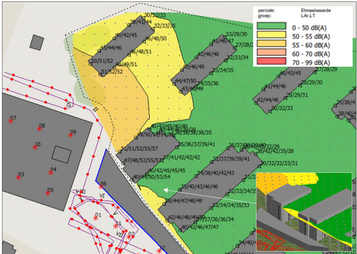
Afbeelding 4.3 Geluidcontour (etmaalwaarde) (beoordelingshoogte 13,5 meter)
