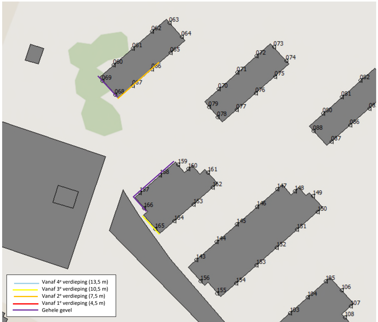
Afbeelding 5.5 Weergave totaal toe te passen dove gevels bij te hoge geluidbelasting (langtijdgemiddelde en maximaal geluidniveau – L_{Ar,LT} / L_{Amax} )
