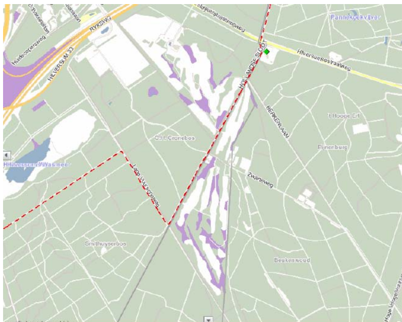
figuur5.2 Globale indicatie van vluchtroutes in de omgeving van de hogedruk aardgasleiding (rode stippellijn) voor locatie 2 (bron: risicokaart, Kadaster)
