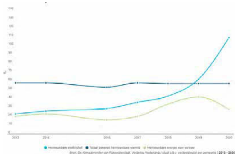
Figuur 6.24 Gebruik hernieuwbare energie (in terra joule) in Den Helder in de periode 2013 - 2020 (Bron: Den Helder in Cijfers op www.denhelder.nl )
