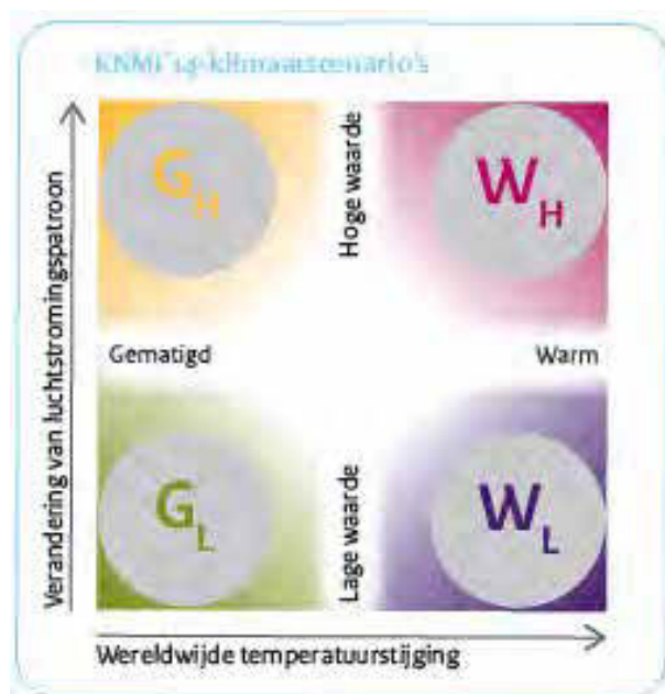
Figuur 4.1. KNMI's vier klimaatscenario's
