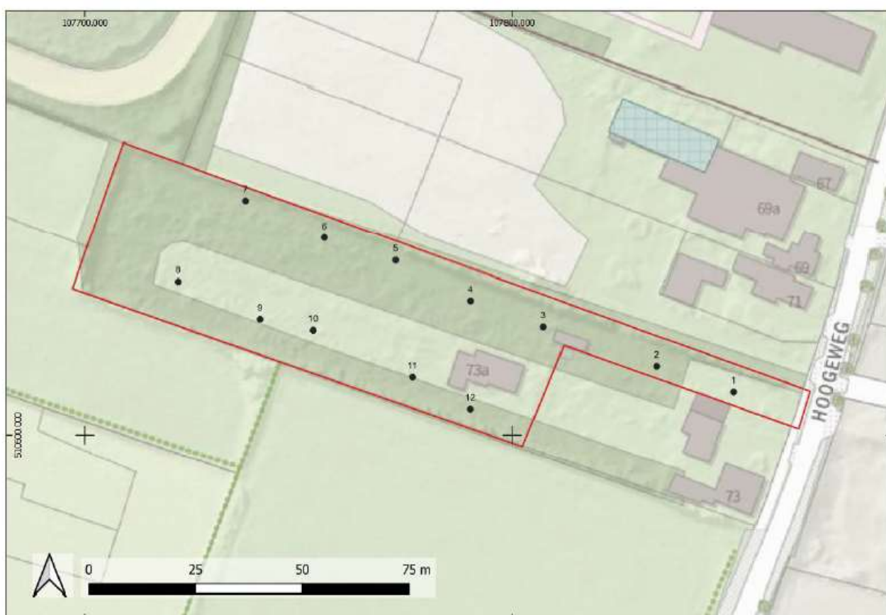
Figuur 3.1. Overzicht boorpunten.
