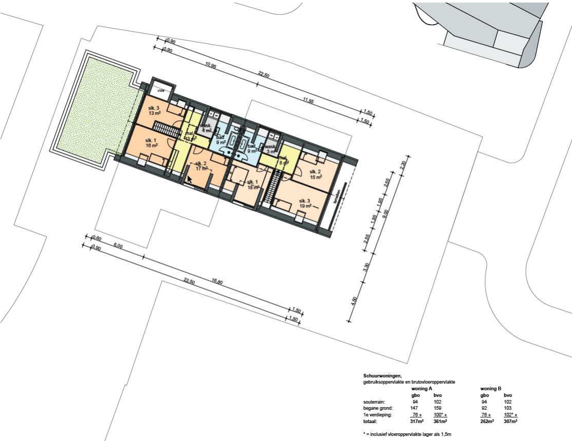
Plattegrond verdieping met voorlopig ontwerp bouwvolumes twee-onder-een-kapwoningen Duin en Vaart 12 (bron: Commandeur Haumann architecten).
