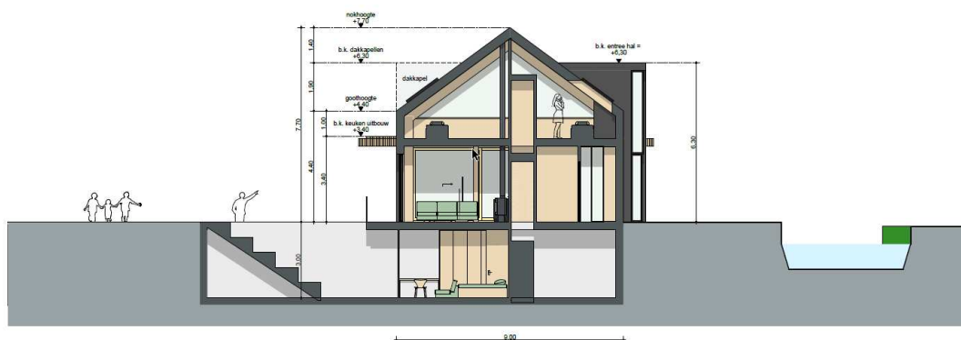
Concept 3d visualisatie dwarsdoorsnede twee-onder-een-kapwoningen Duin en Vaart 12 (bron: Commandeur Haumann architecten).
