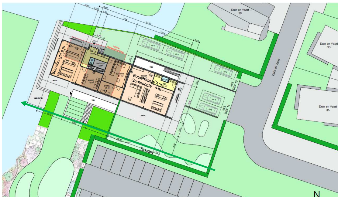
Plattegrond met voorlopig ontwerp bouwvolumes twee-onder-een-kapwoningen Duin en Vaart 12 (bron: Commandeur Haumann architecten).
