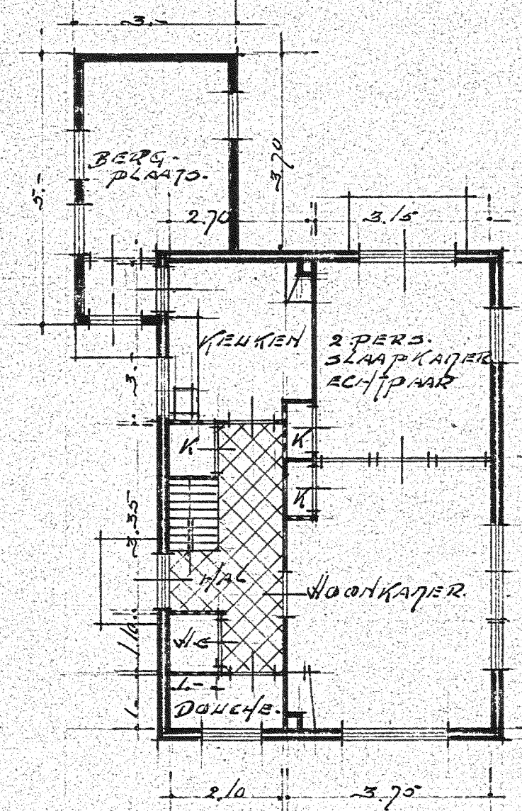
BEGANE GROND.
