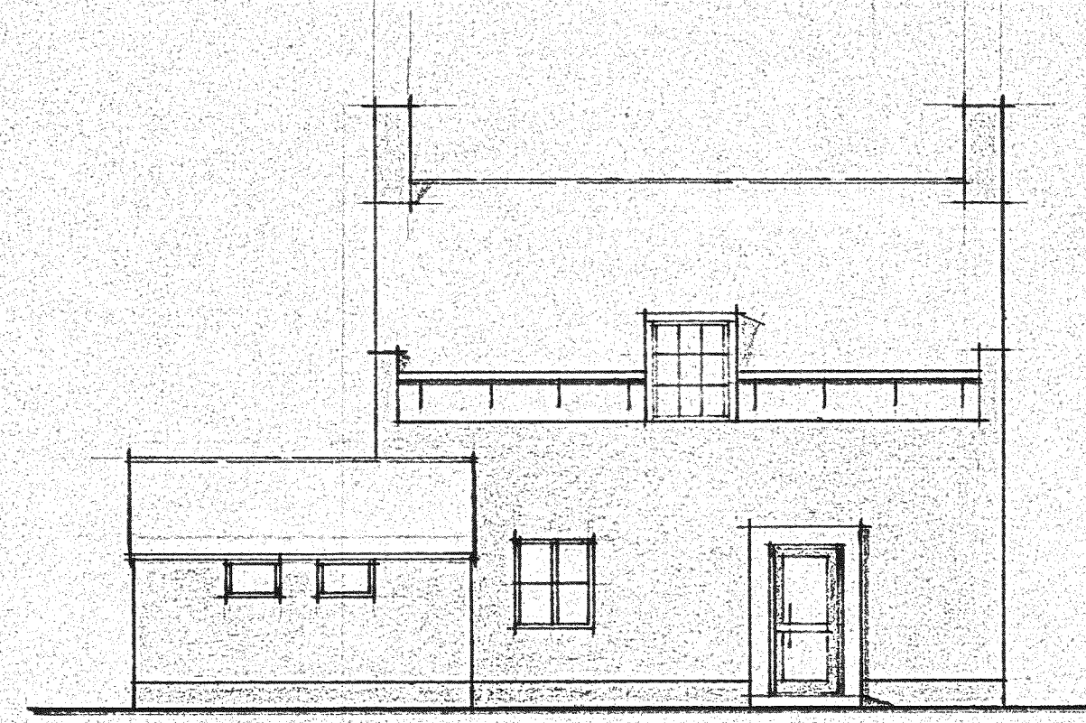
NOORDGEVEH.
