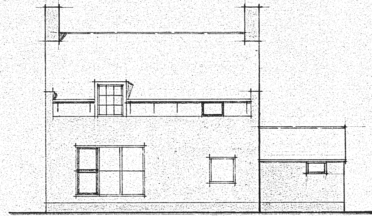
ZUIDGEVEH.
