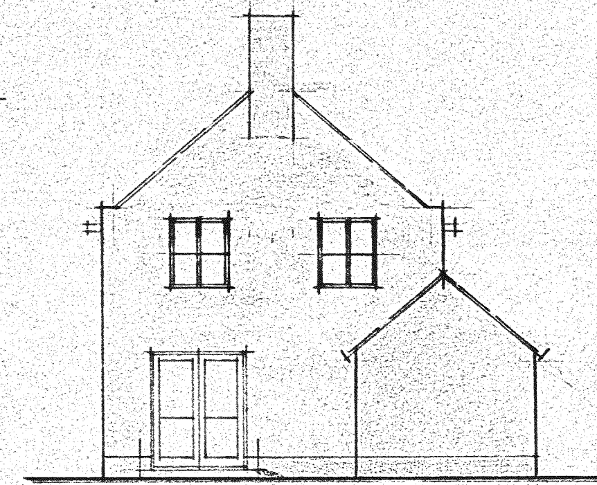
OOSTGEVEH.
