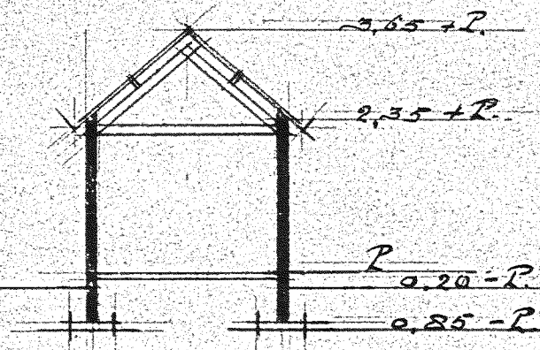
DOORSNEDEN BERGPLAATS
