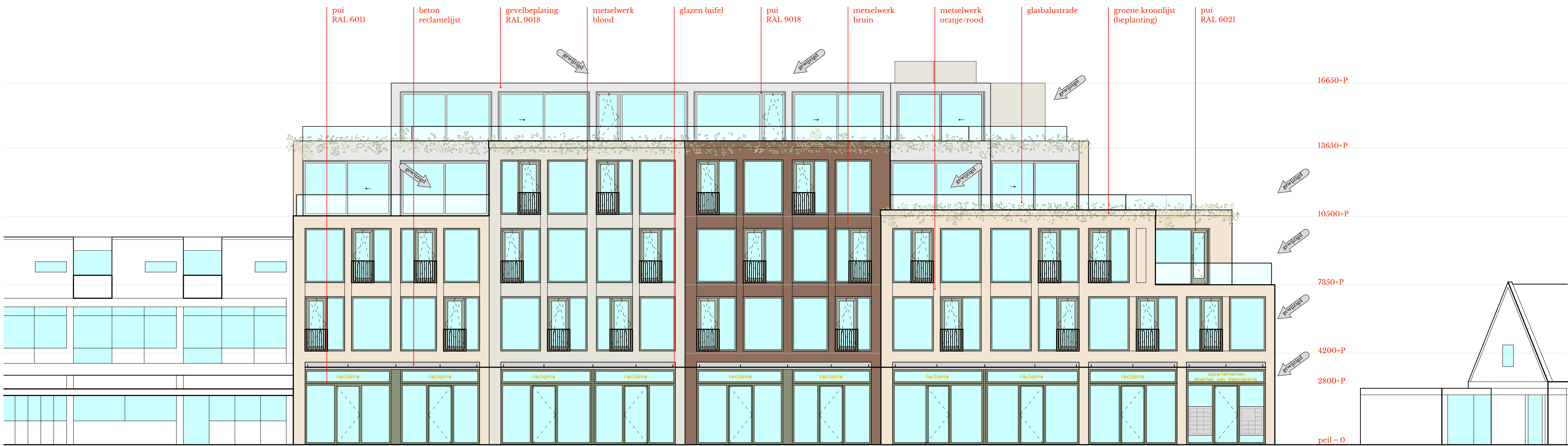
voorgevel
