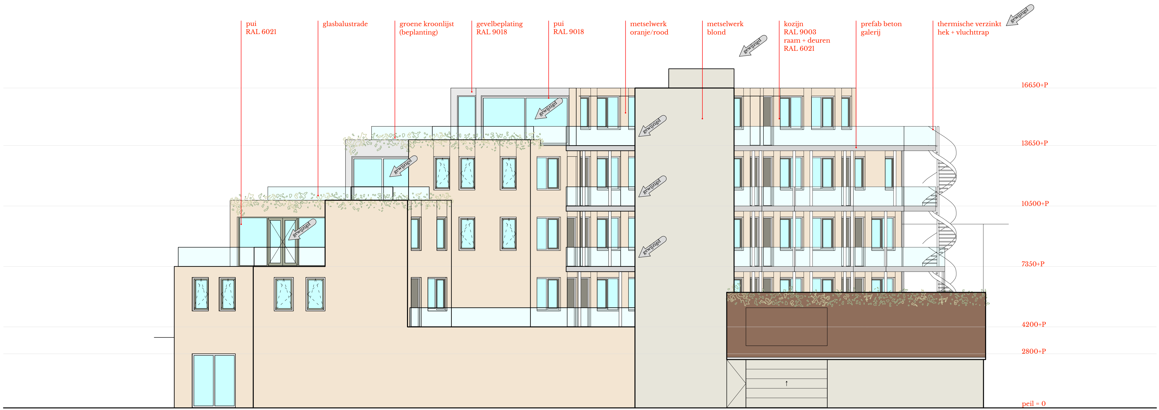
rechterzijgevel
