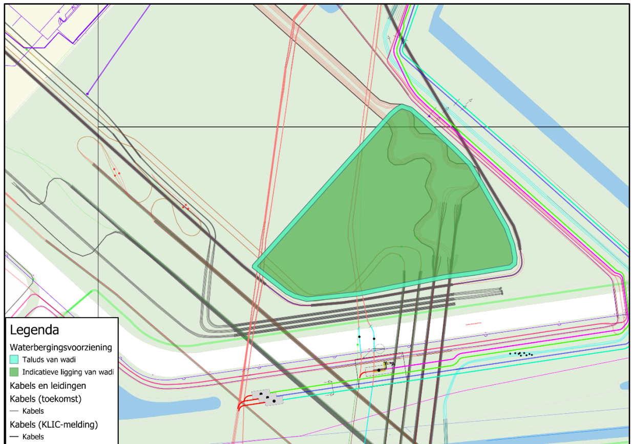
Figuur 10: Indicatieve ligging van wadi binnen gebied B.
