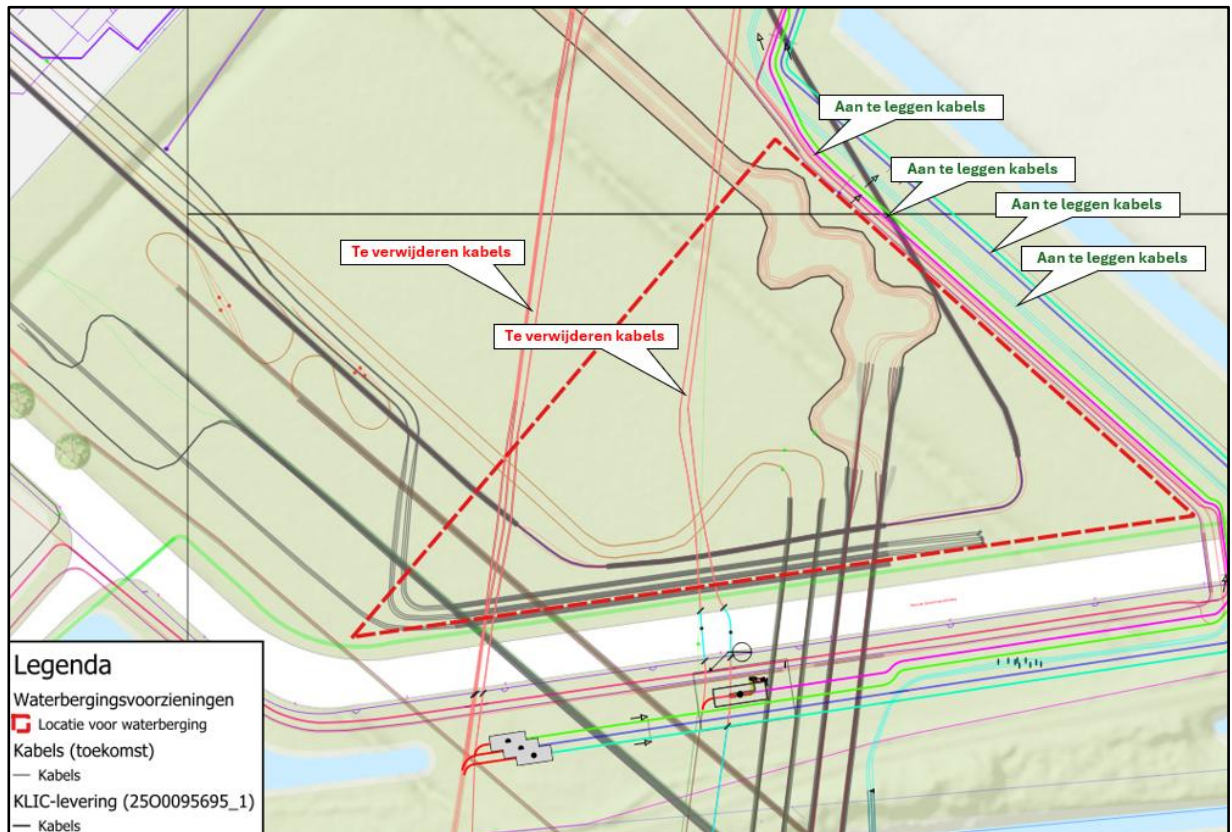
Figuur 8: Ligging van bestaande en nieuwe kabels in kansrijke gebied B.
