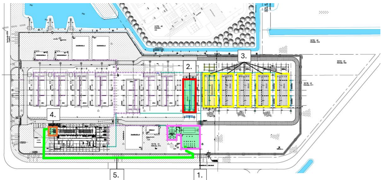
Figuur 4-2 Toekomstige situatie hoogspanningsstation Vijfhuizen
