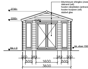
Vooraanzicht
