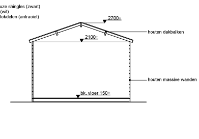
Doorsnede A-A
