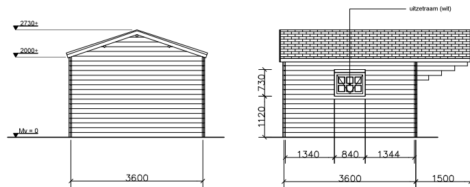
Achteraanzicht
