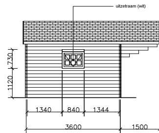
Linkerzij aanzicht
