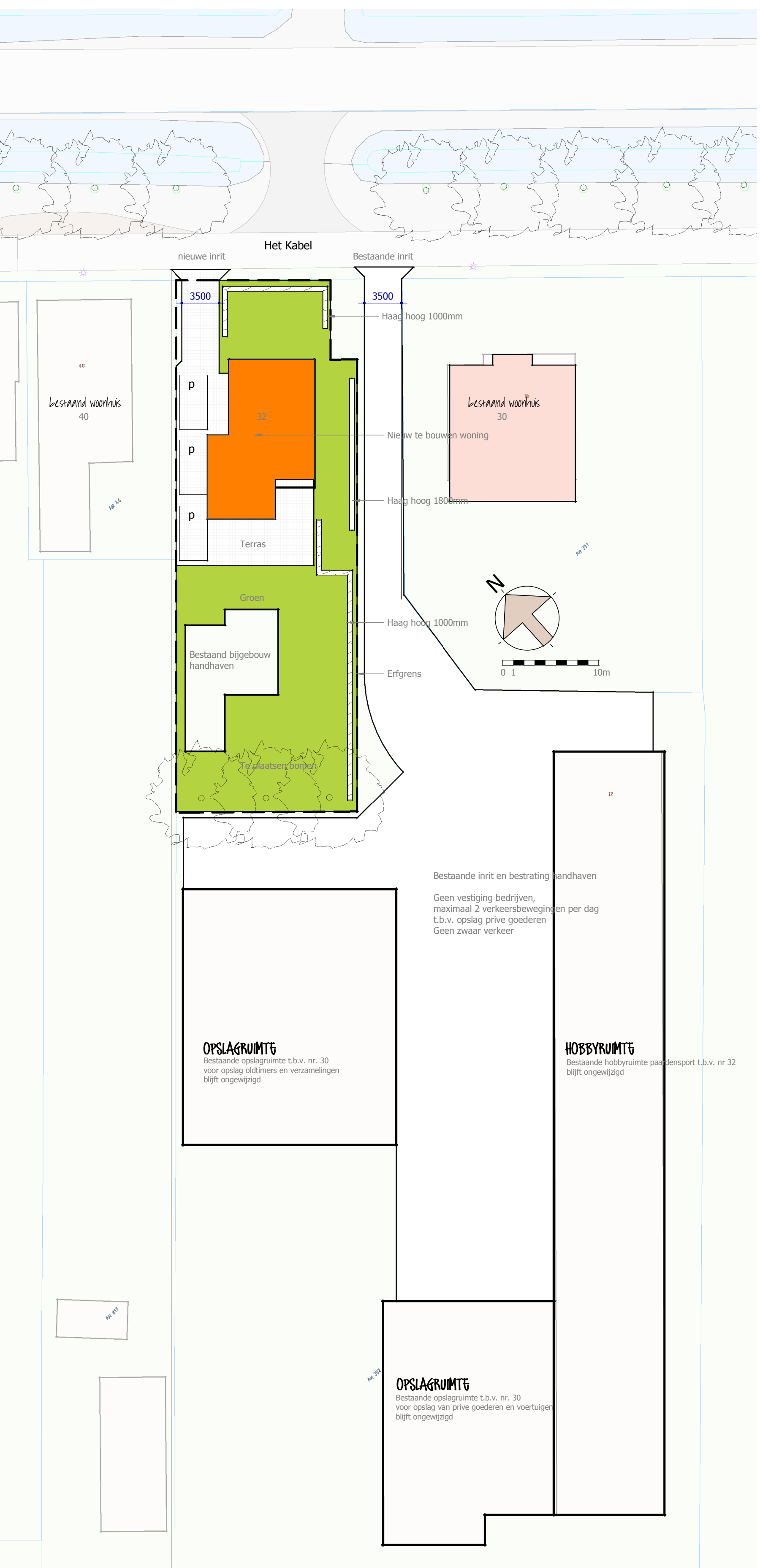
1 | terreinplan nieuw 1 : 300
