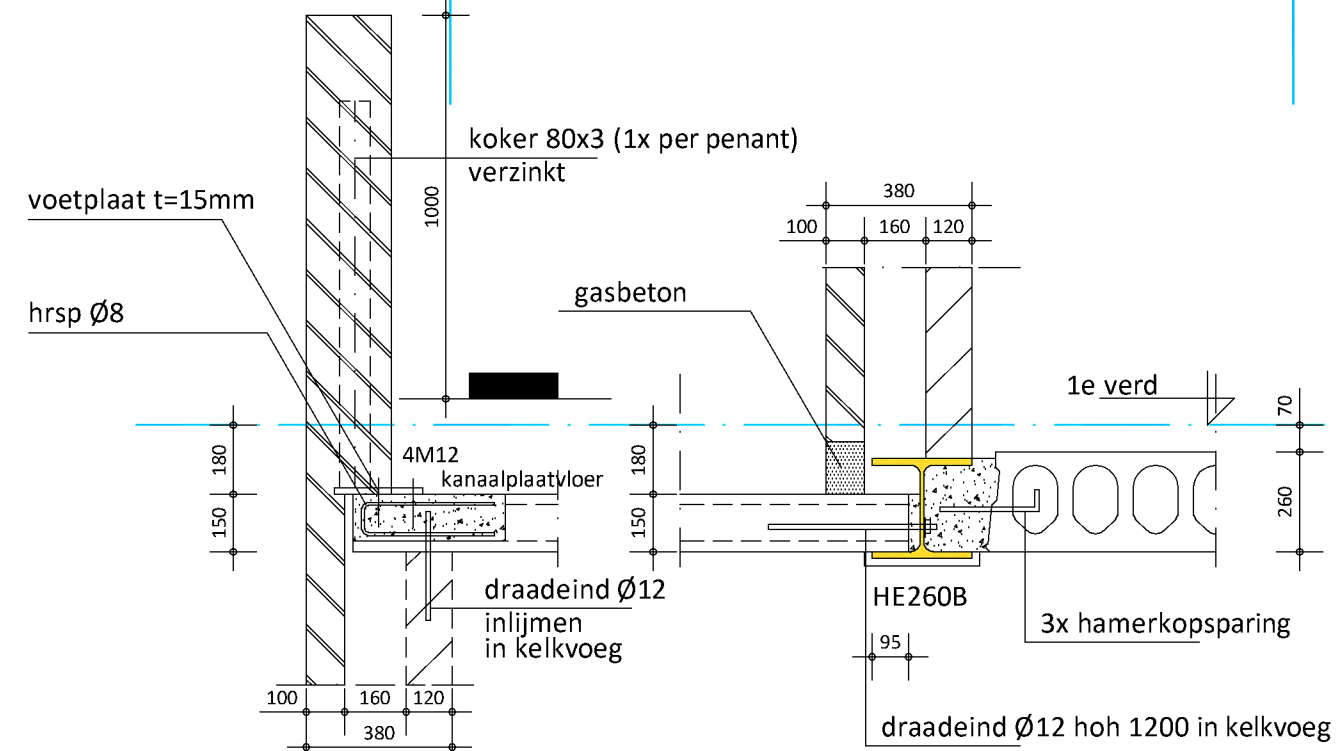
det 1.2
