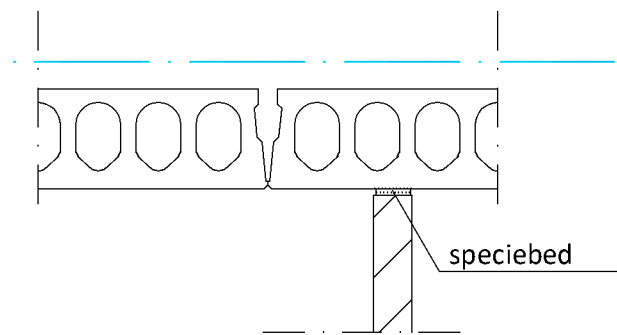
det 1.4
