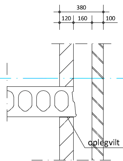
det 1.5
