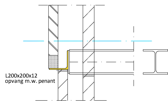
det 1.6
