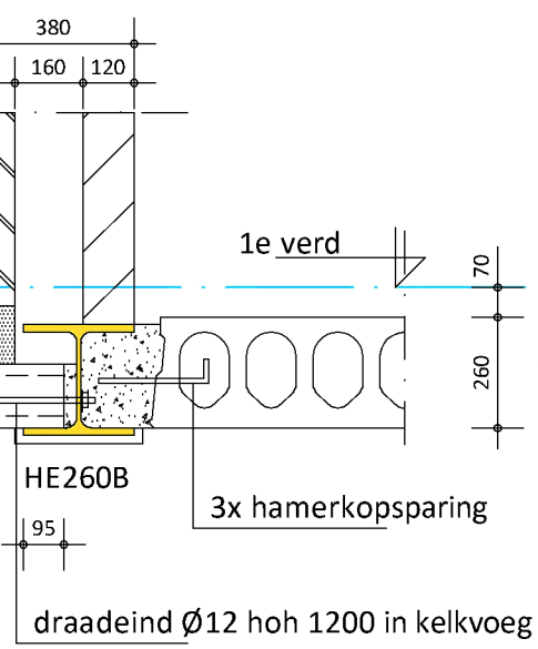
det 1.3
