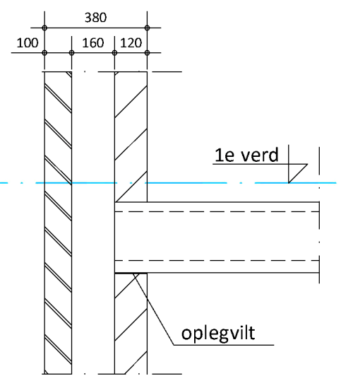
det 1.1
