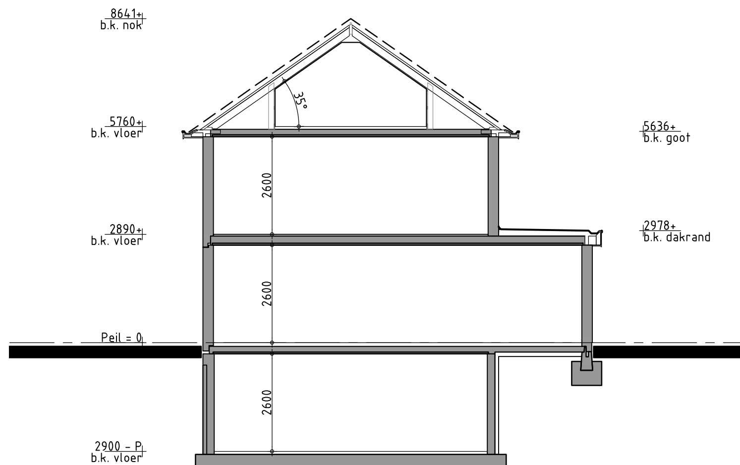
Snede A-A
