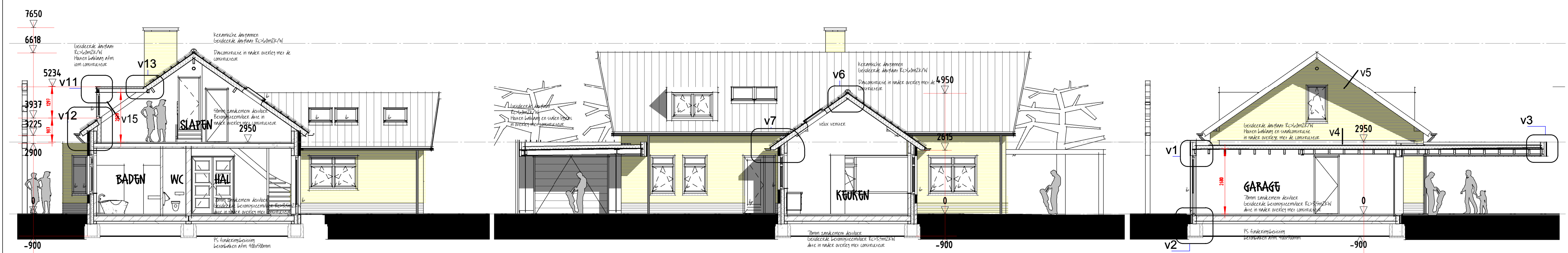
6 DOORSNED E B 1 : 100
