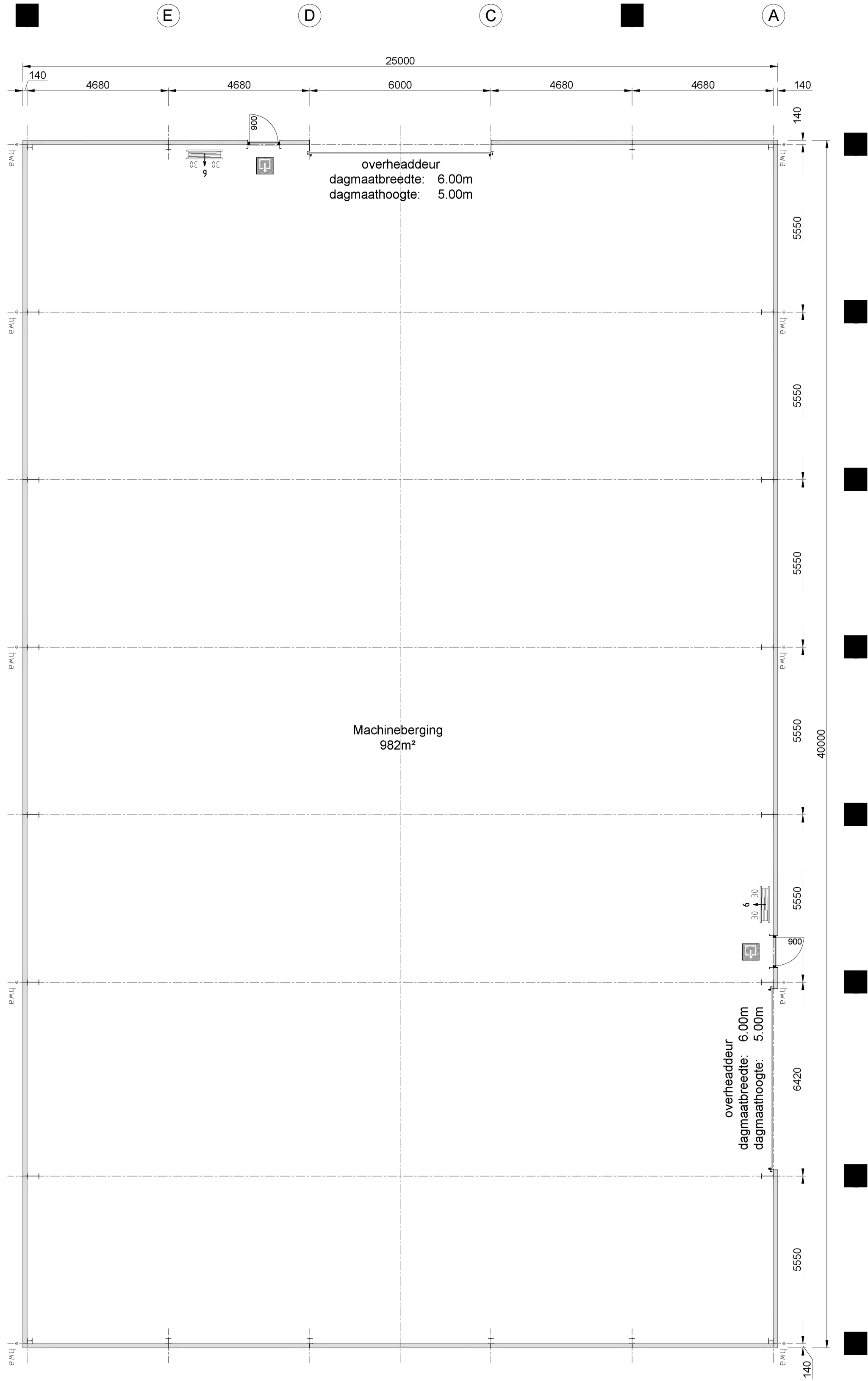
Plattegrond
