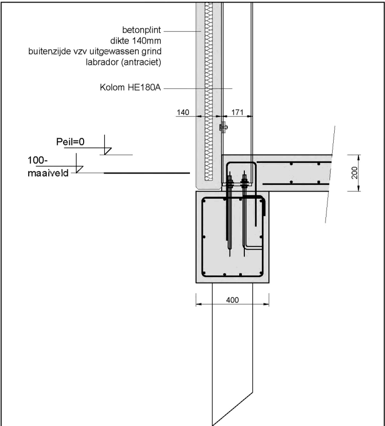
Doorsnede II
