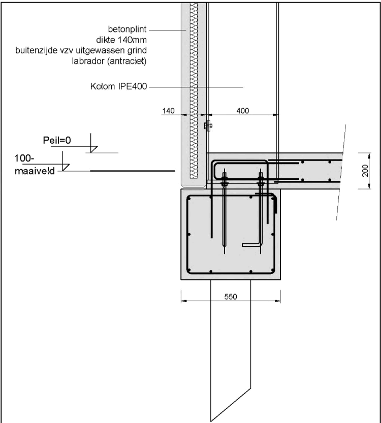
Doorsnede I
