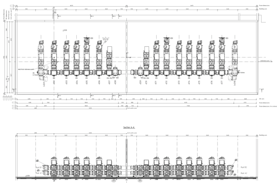
Figuur 3: Bovenaanzicht en zijaanzicht gelijkende 150kV GIS-installatie (van OS Velsen, veldindeling wijkt af)
